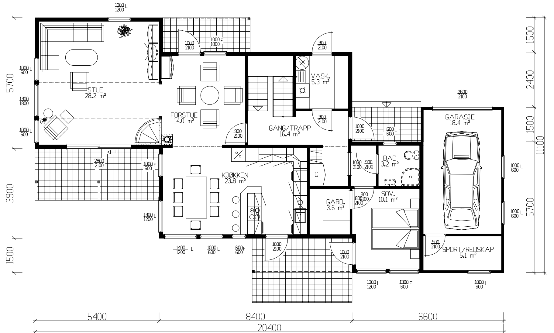
HOVEDPLAN 108,1m² BRA + GARASJE 23,5m² BRA
