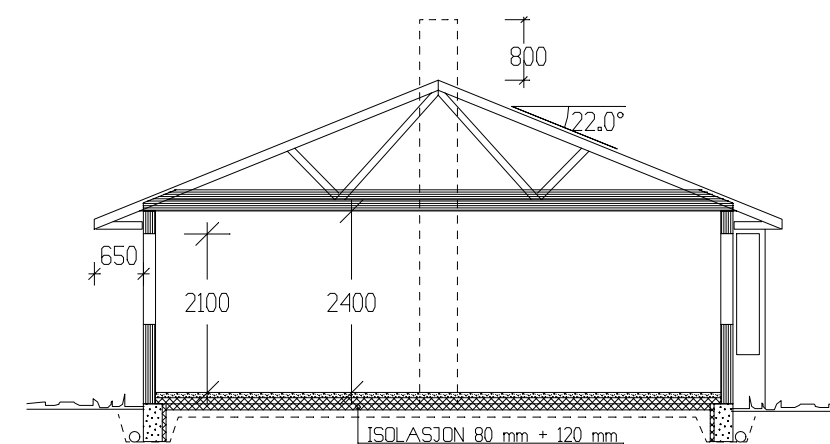
SNITT
