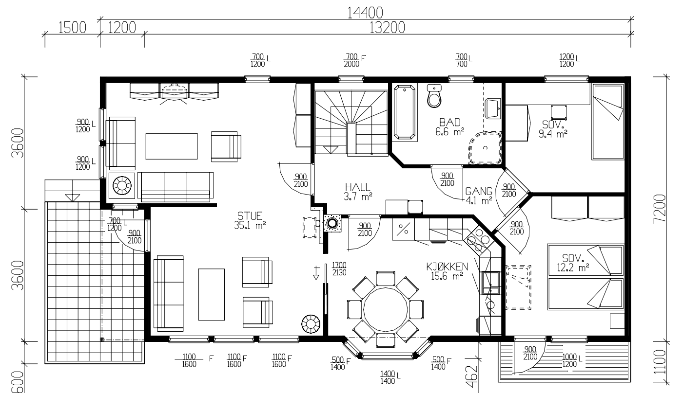
HOVEDPLAN 93.4 m² BRA-K
