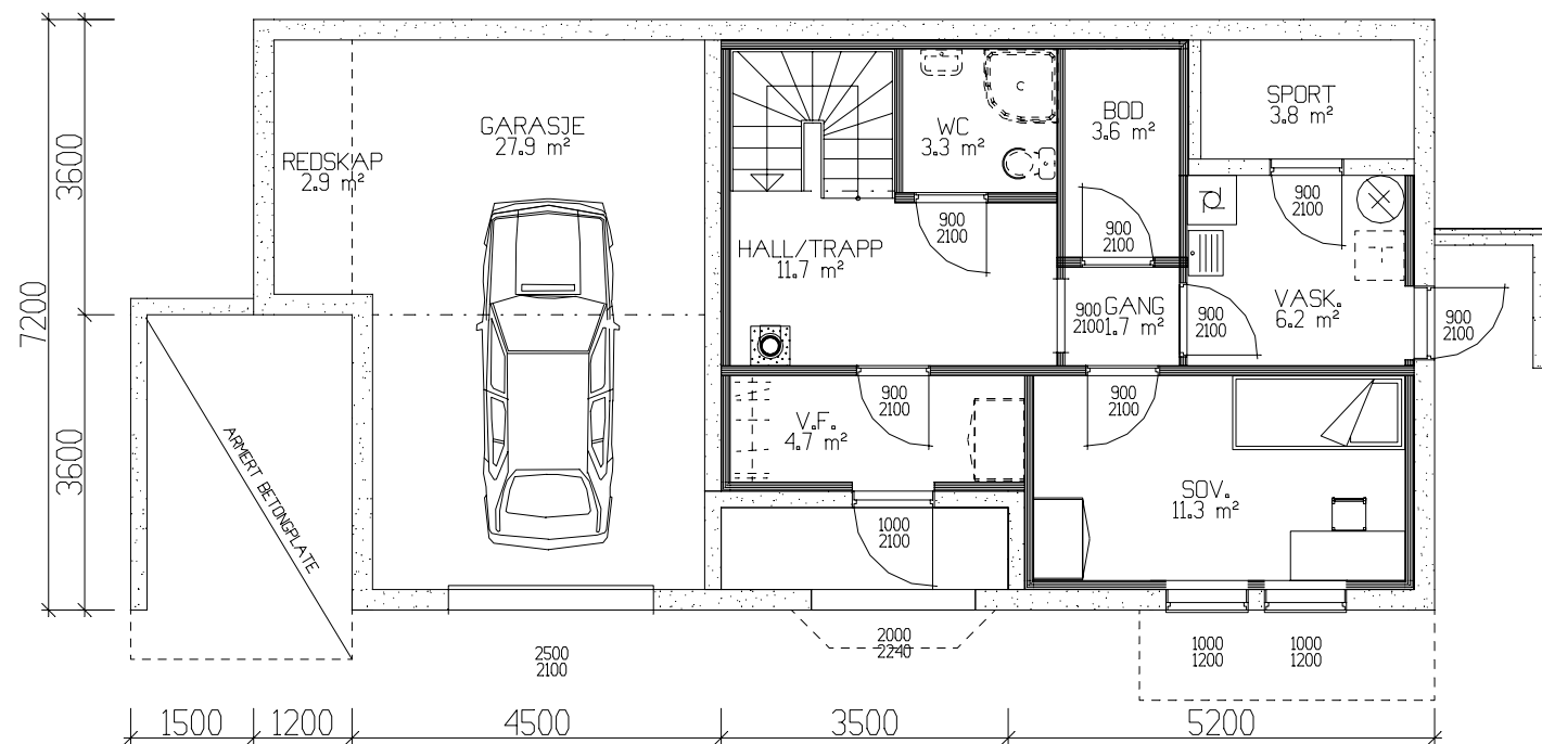
UNDERETASJE 45.6 m² BRA-K, + sport 6.7 m² BRA.
