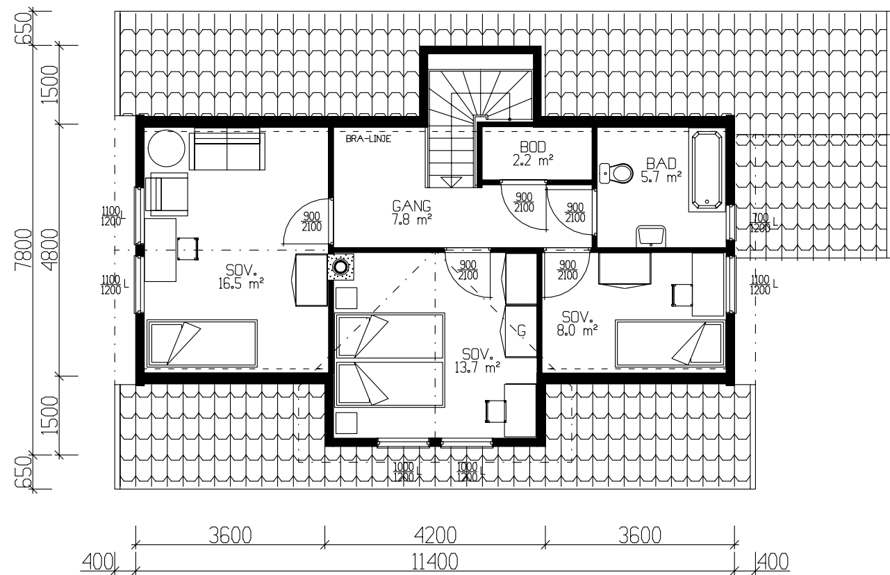
LOFTSPLAN 55.6m² BRA-K
