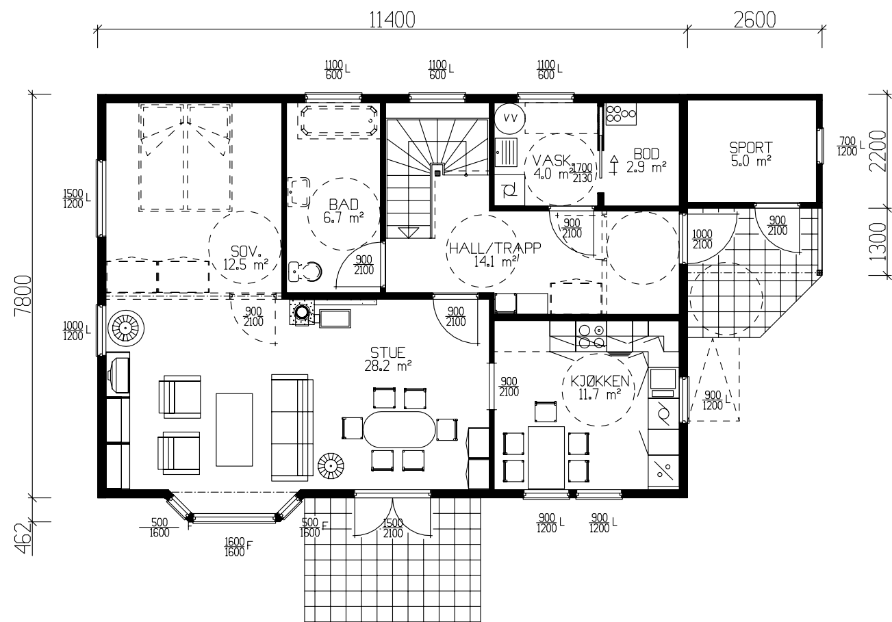
HOVEDPLAN 83.8m² BRA-K + BOD 5.0m²
