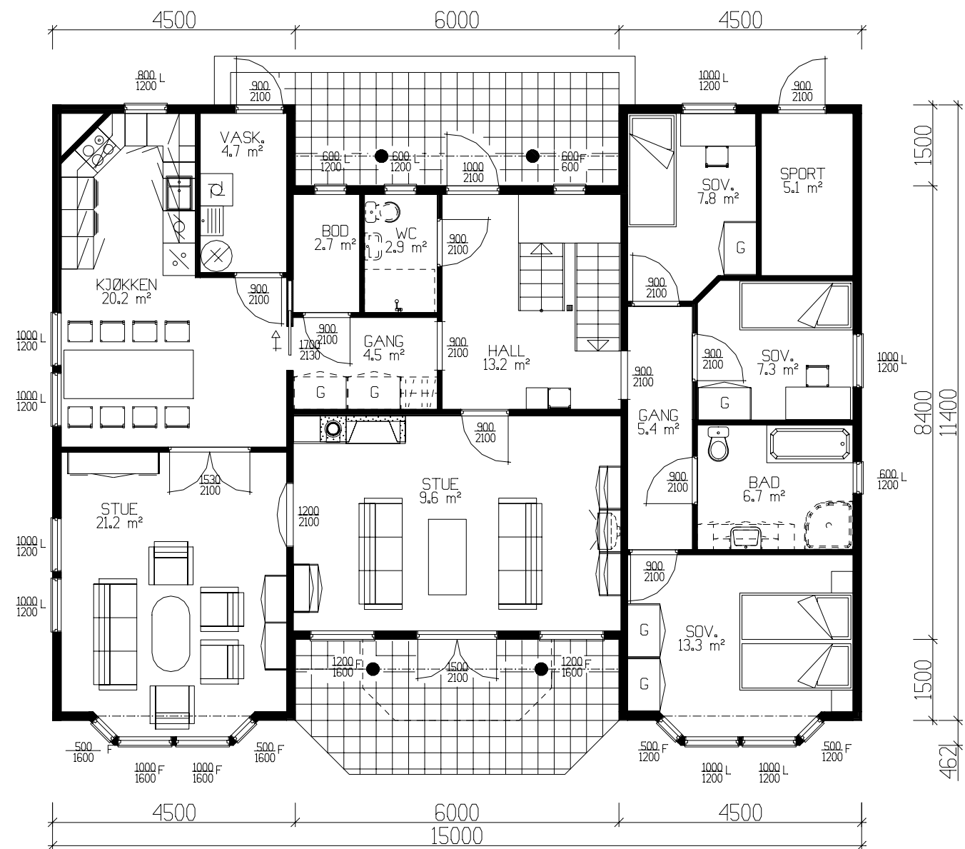
HOVEDPLAN 145.5m² BRA
