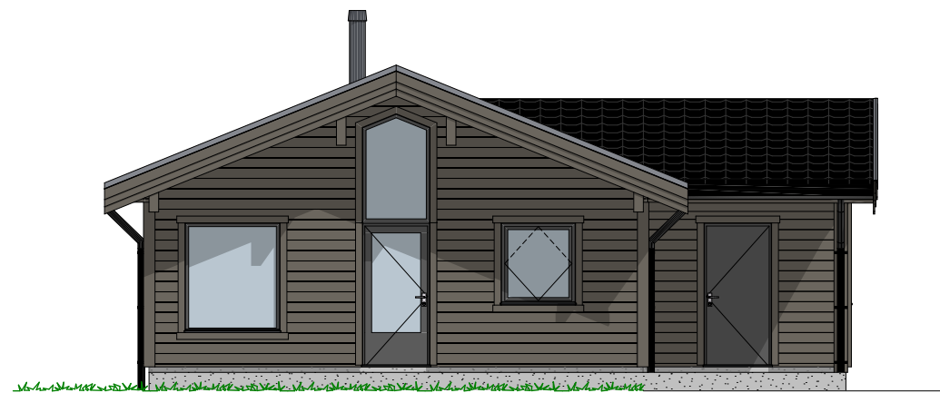
1:100 Fasade Vest
