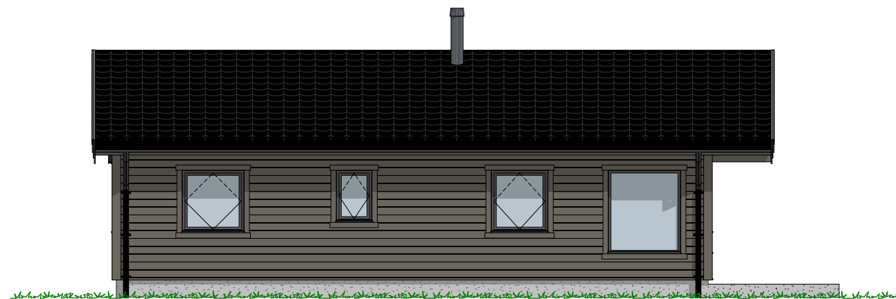
1:100 Fasade Nord
