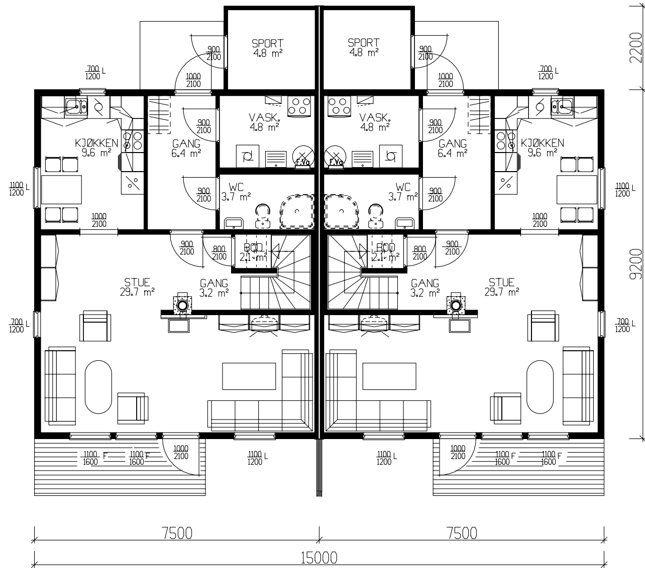
HOVEDPLAN - 2 LEILIGHETER a 64,1m² BRA
