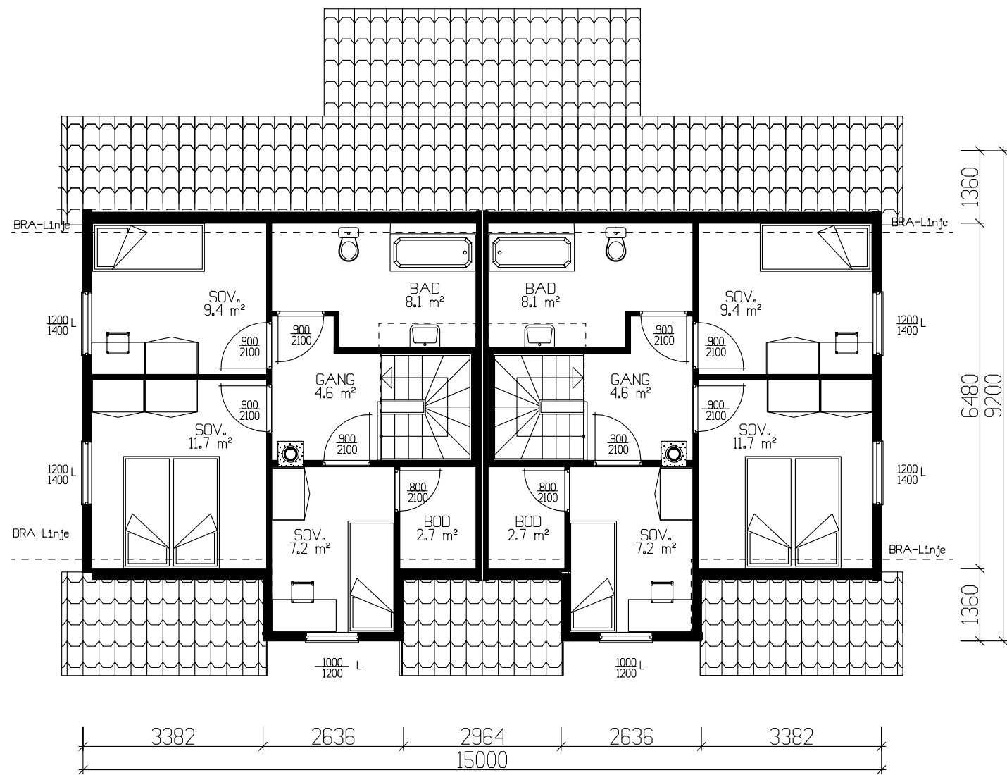
ETASJEPLAN - 2 LEILIGHETER a 47,4 m² BRA
