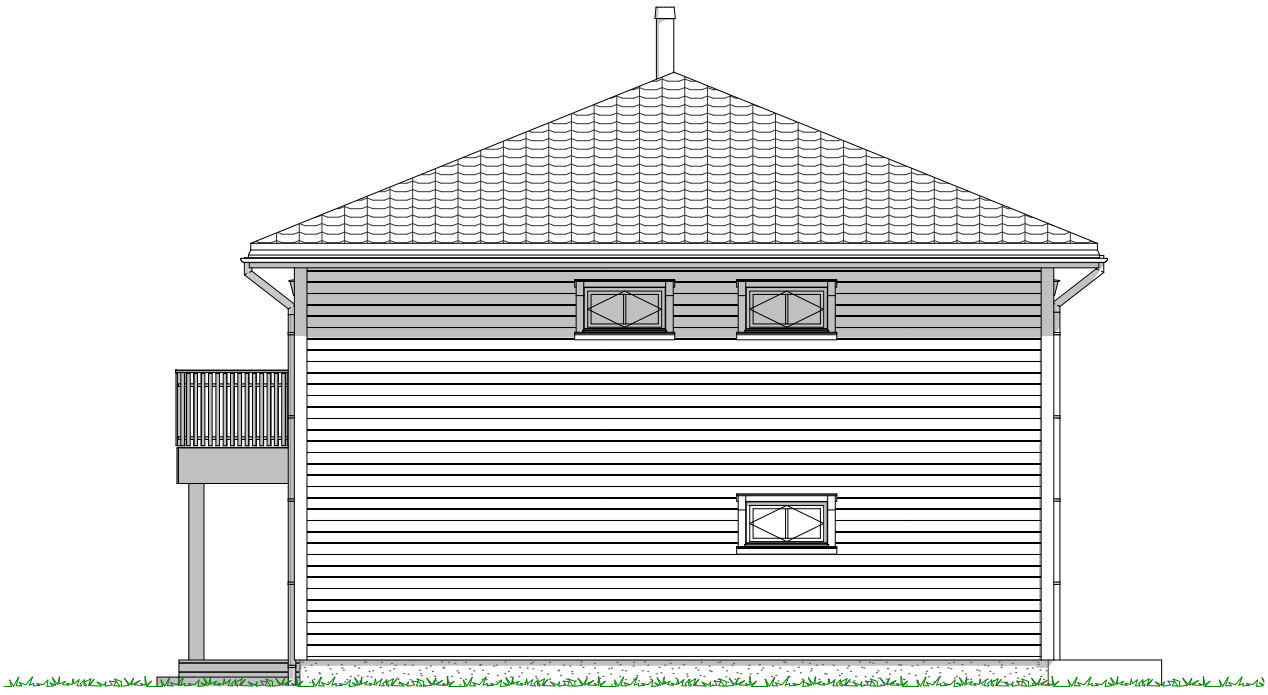
1:100 Fasade Øst
