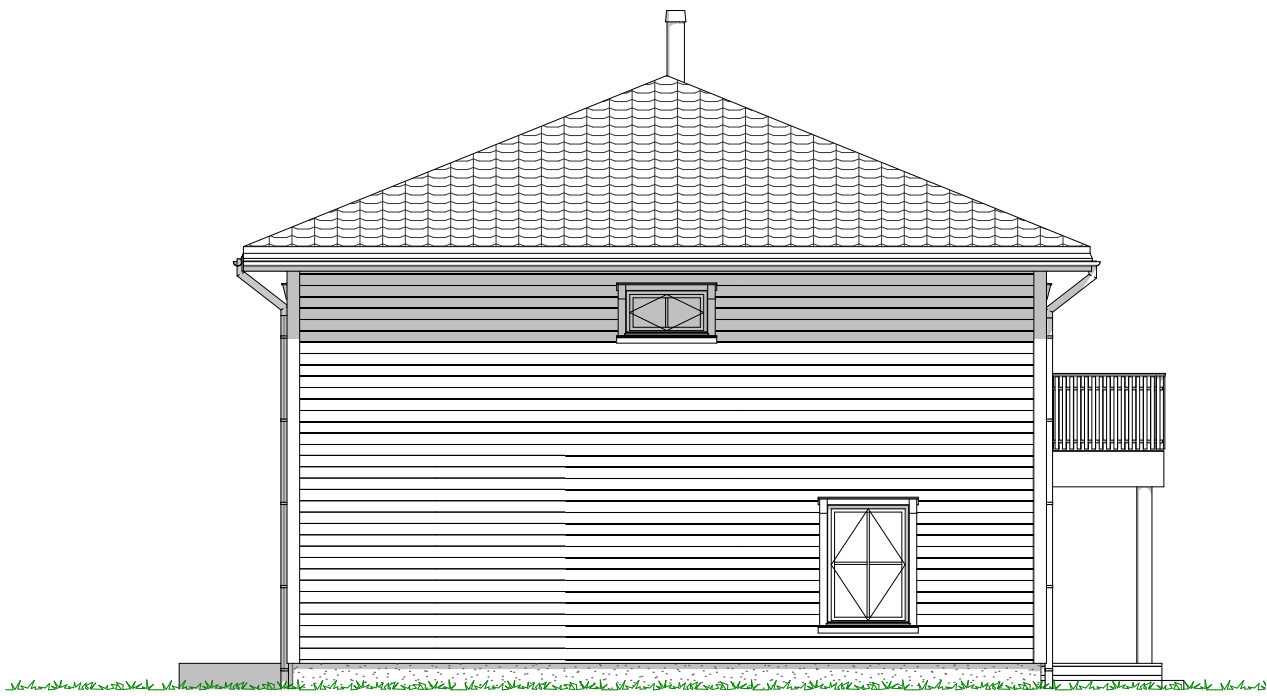
1:100 Fasade Vest
