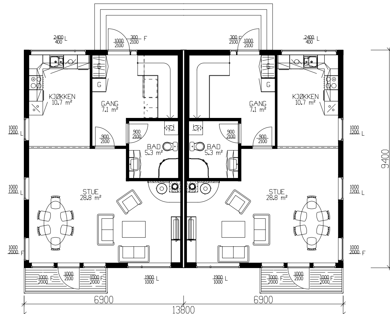
HOVEDPLAN 58,4m² BRA PR. LEILIGHET
