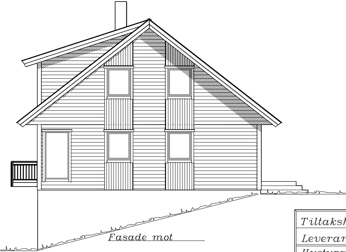
Fasade mot
