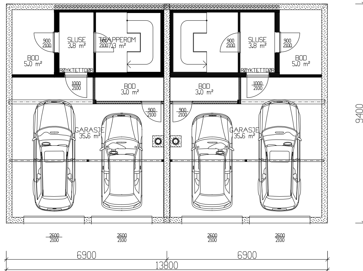
UNDERETASJE 57,2m² BRA
