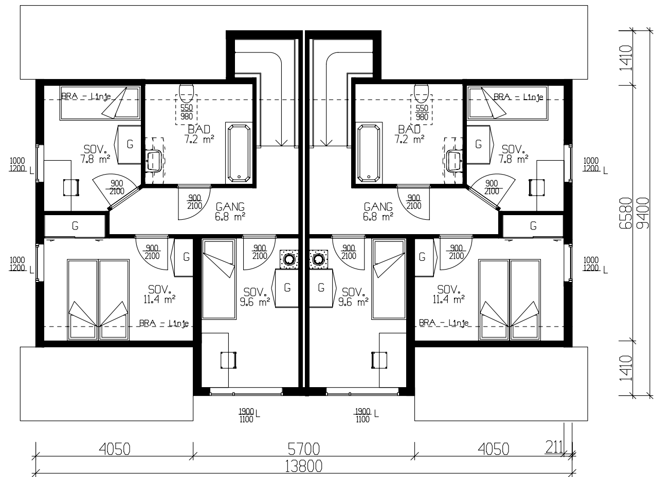
ETASJEPLAN 42,2m² BRA PR LEILIGHET
