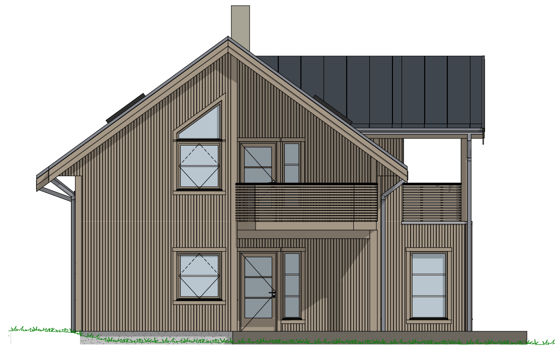
1:100 Fasade NordVest
