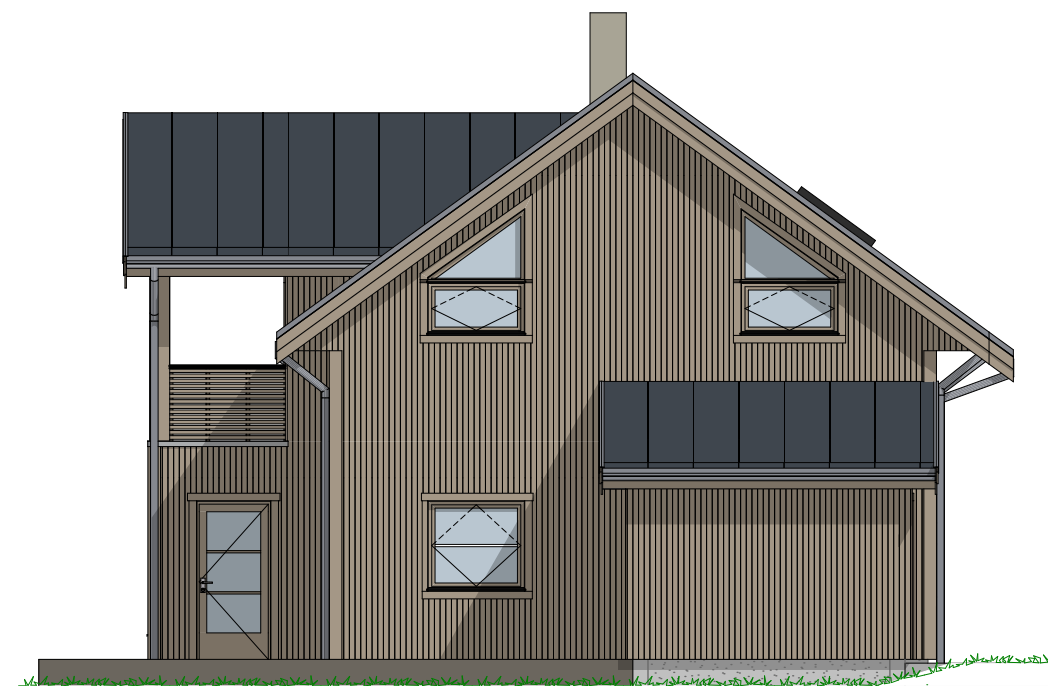
1:100 Fasade SørØst
