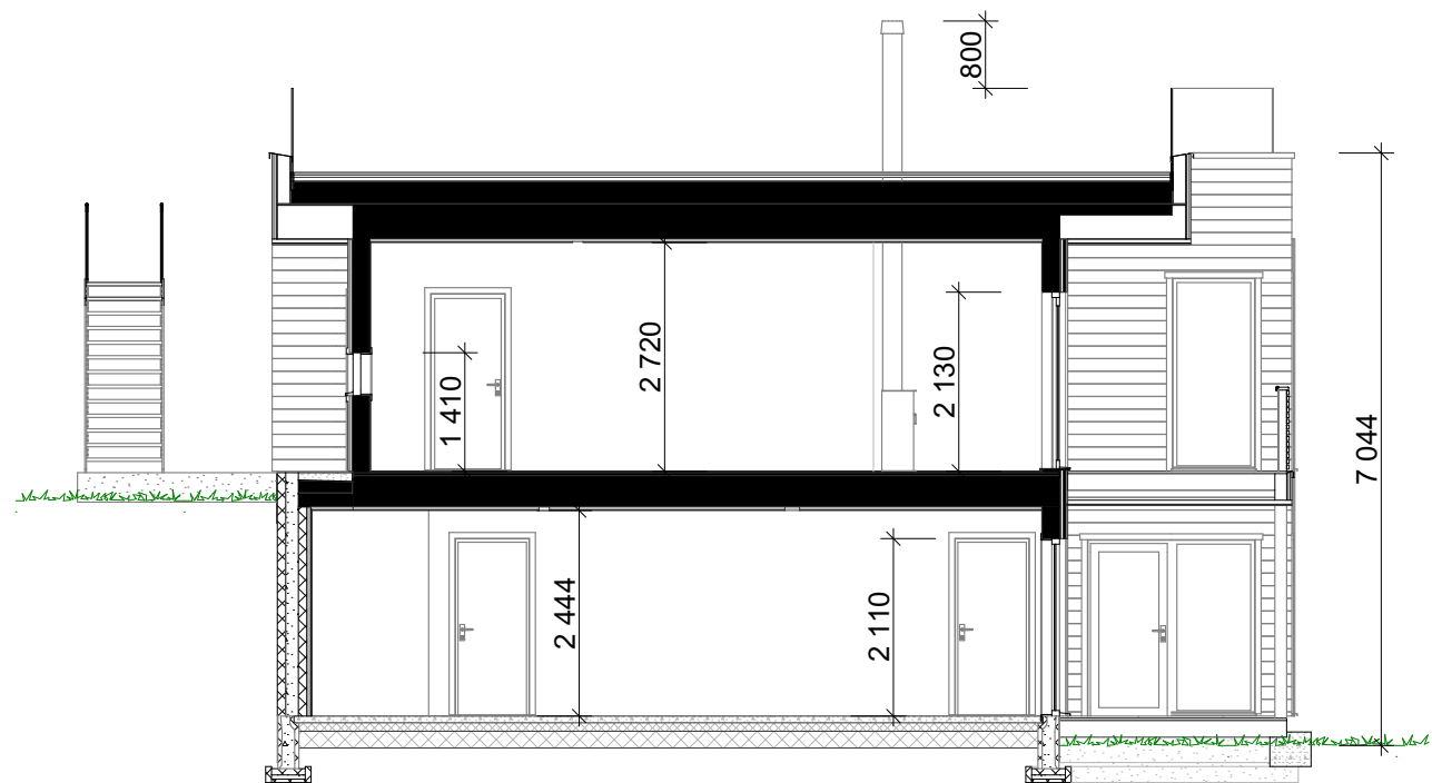
1:100 Snitt A
