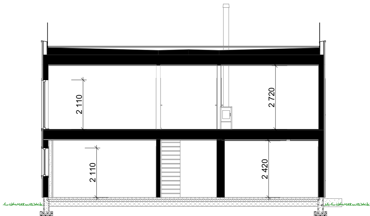
1:100 Snitt B
