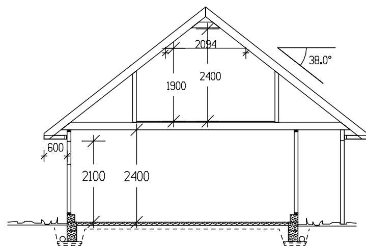
SNITT
