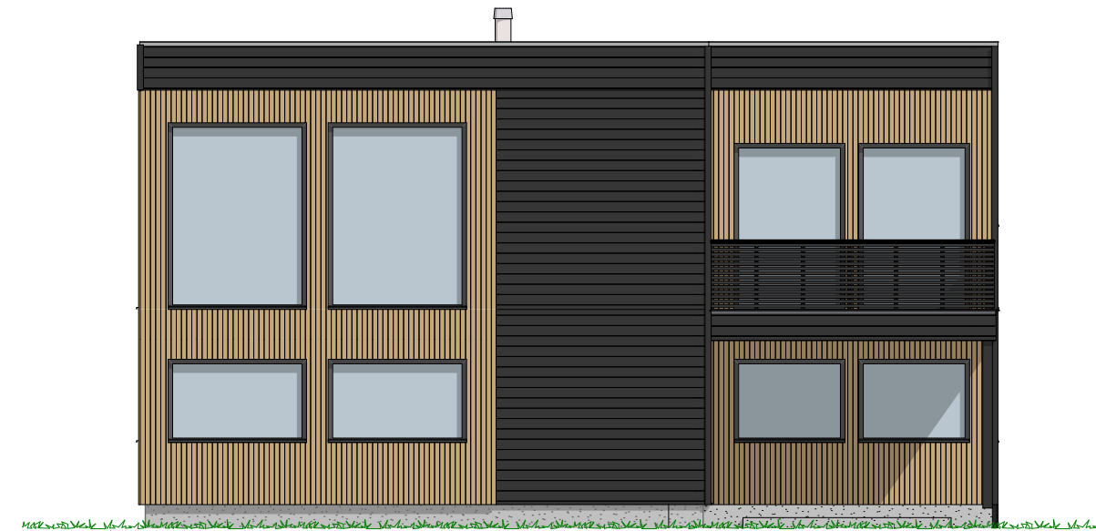
1:100 Fasade Sør
