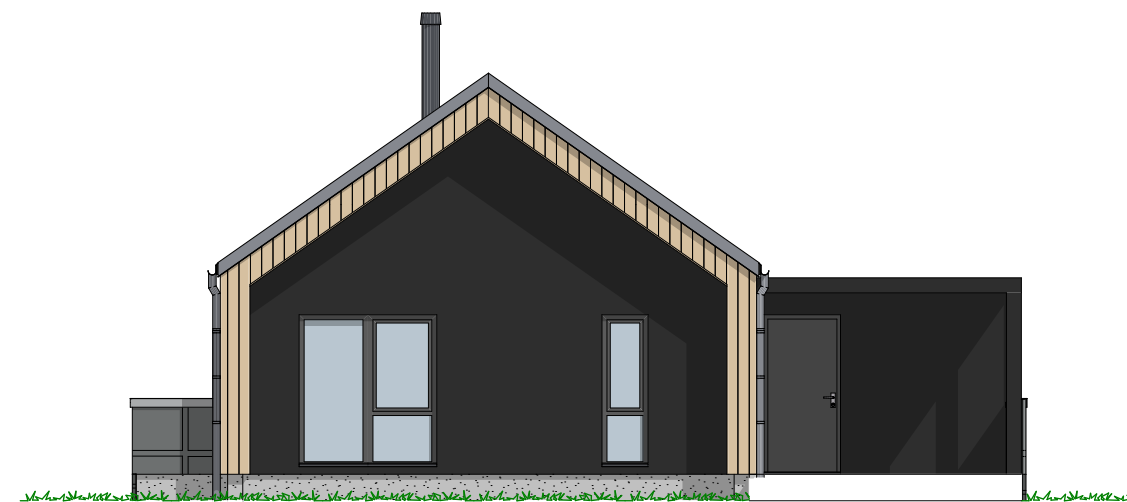
1:100 Fasade Nord
