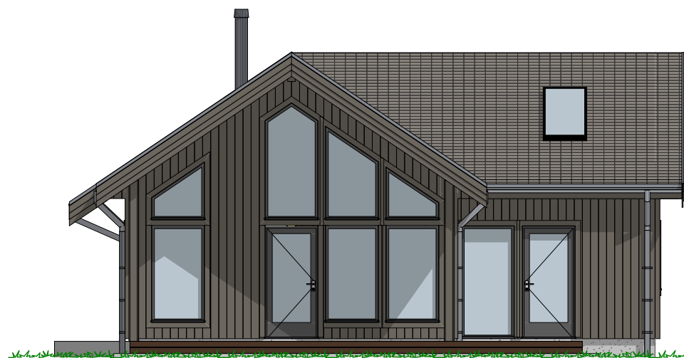
1:100 Fasade Vest
