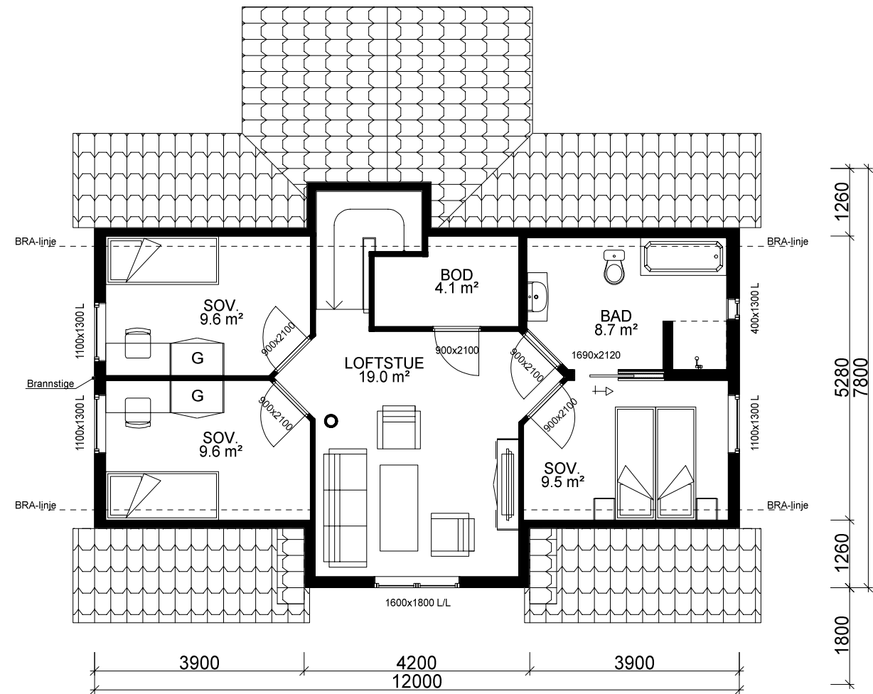
ETASJEPLAN LOFT: 61,5 m² BRA.
