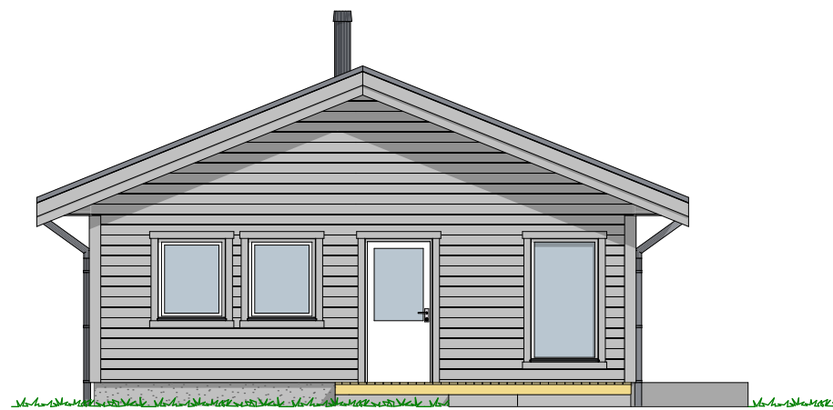
1:100 Fasade Nord
