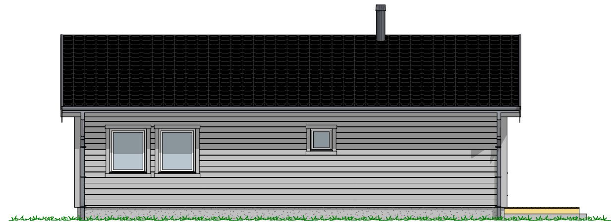
1:100 Fasade Øst
