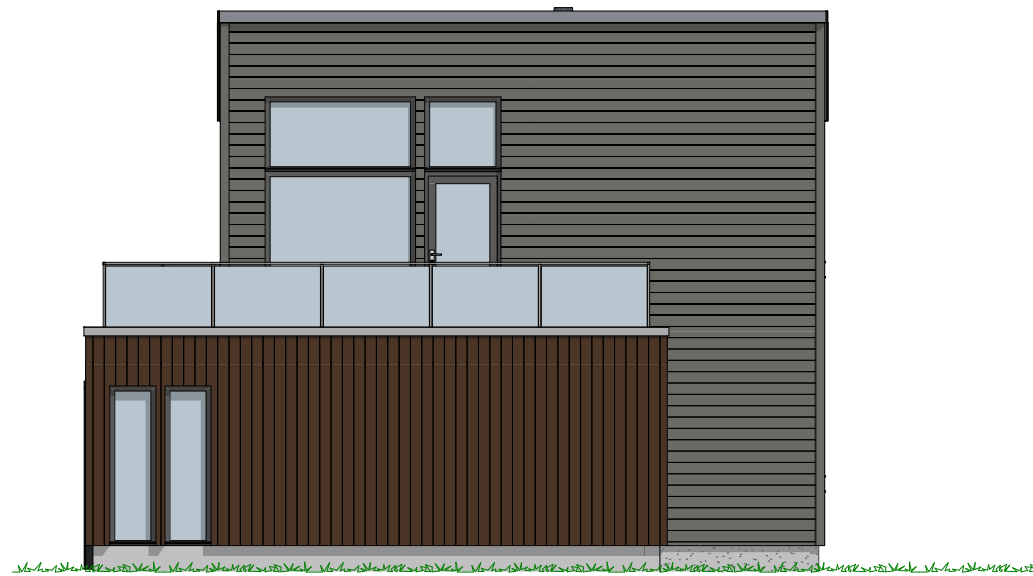
1:100 Fasade NordØst
