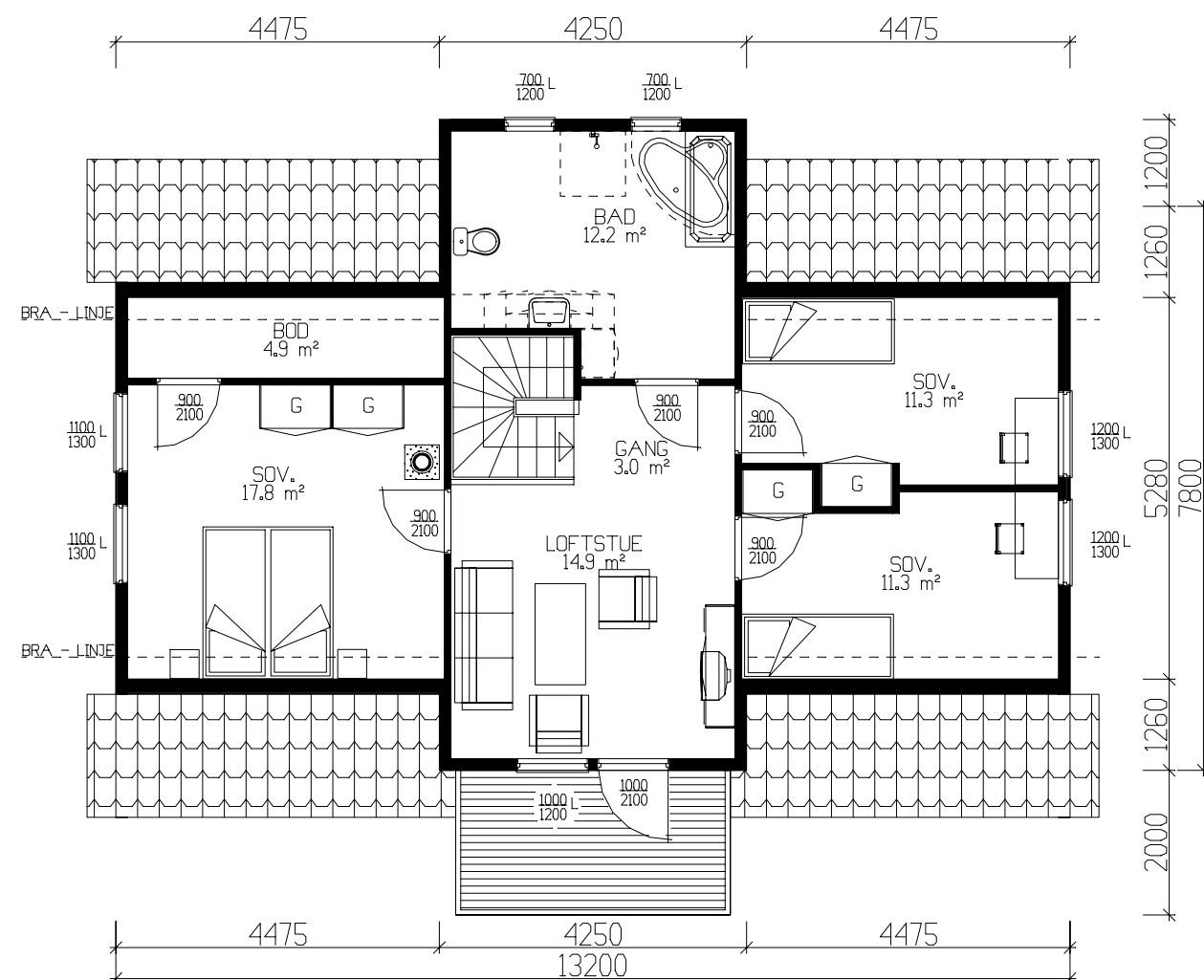
ETASJEPLAN 75.9m² BRA
