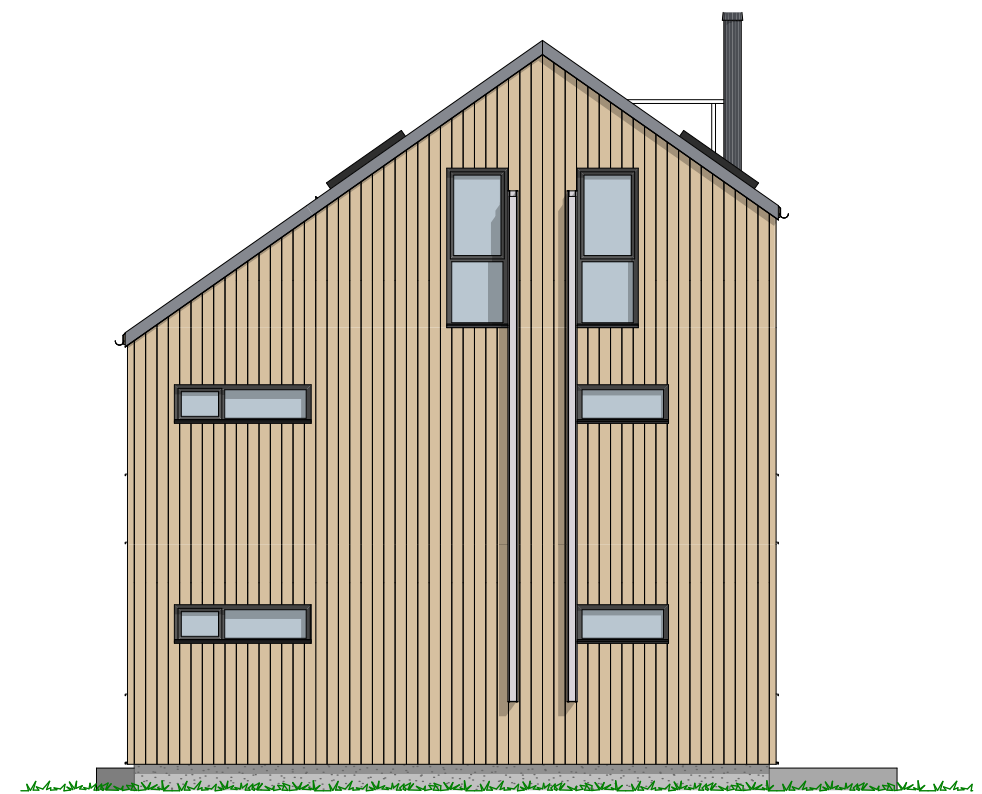
1:100 Fasade Nord
