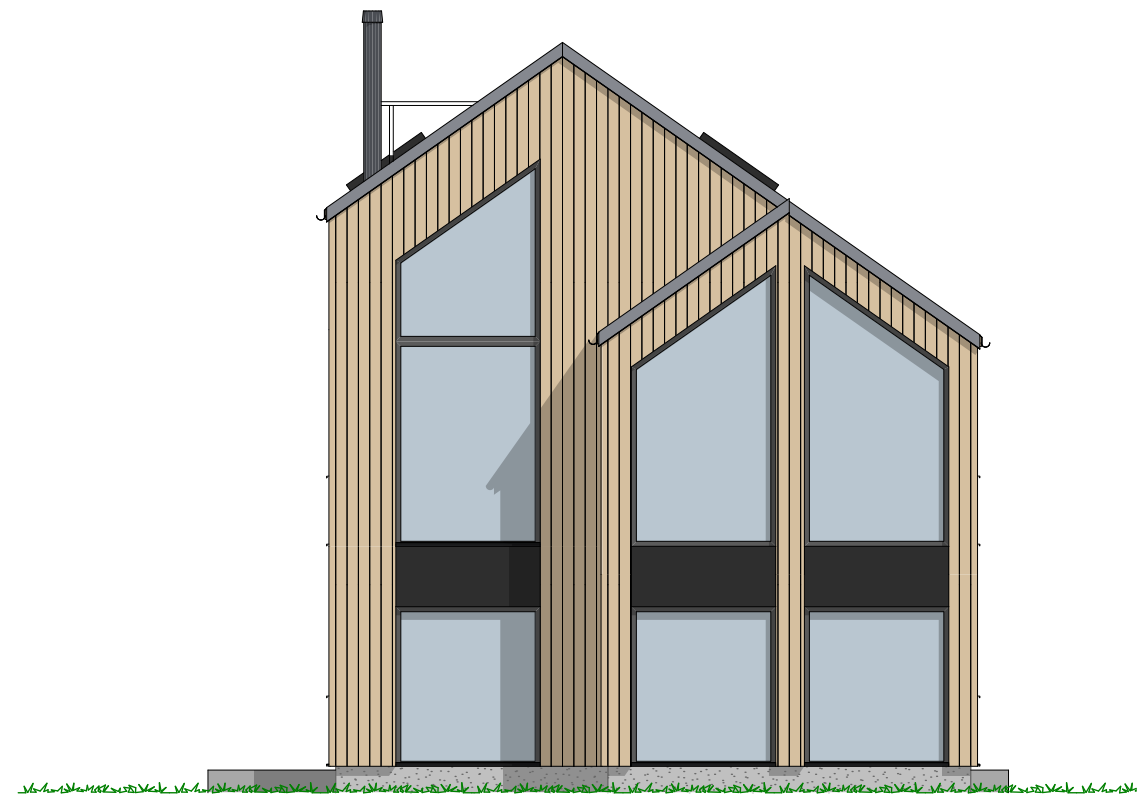
1:100 Fasade Sør
