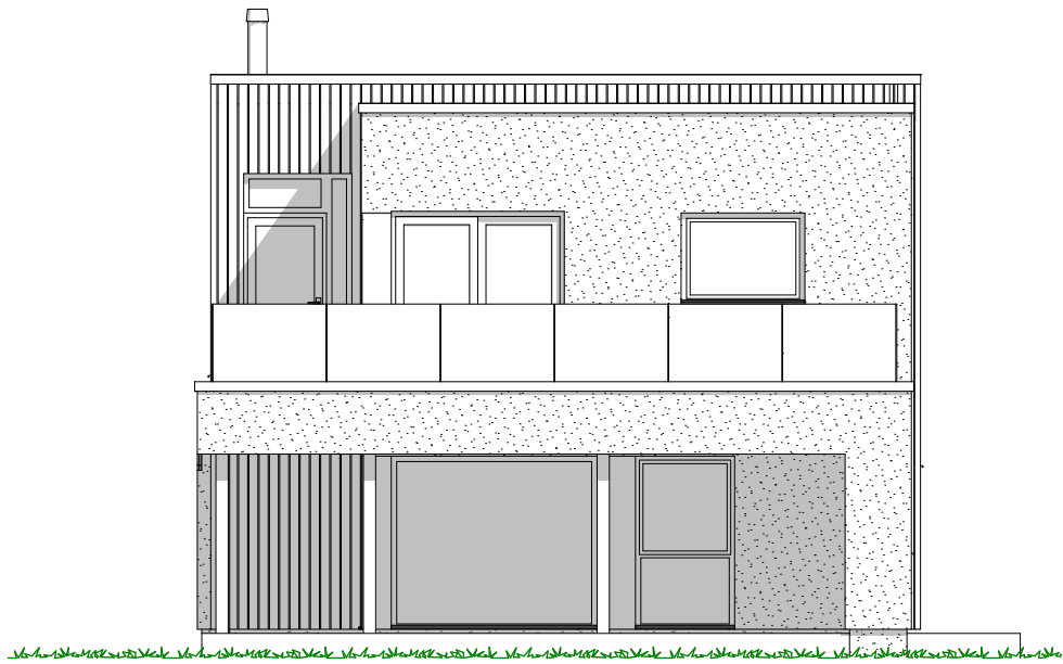
1:100 Fasade sør
