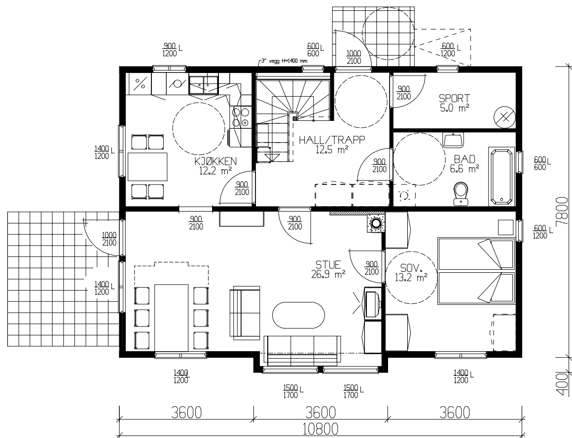
HOVEDPLAN 74.7m² BRA-K + SPORT 5.0m² BRA.
