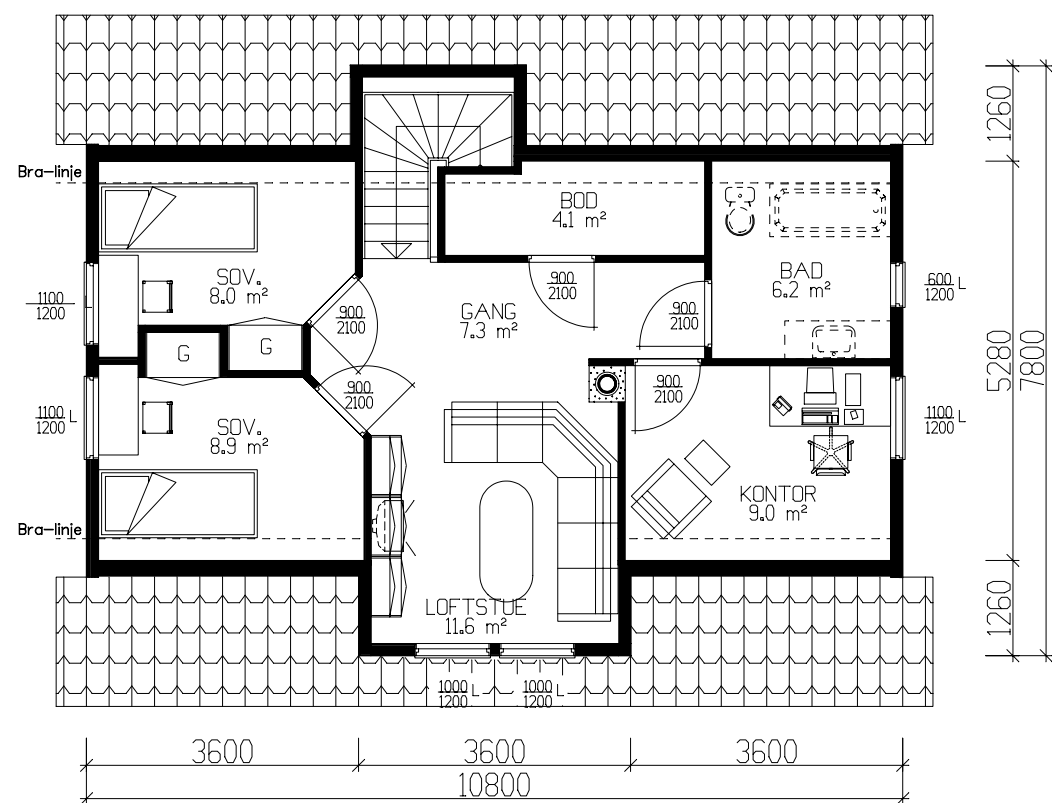
ETASJEPLAN 53.9m² BRA-K
