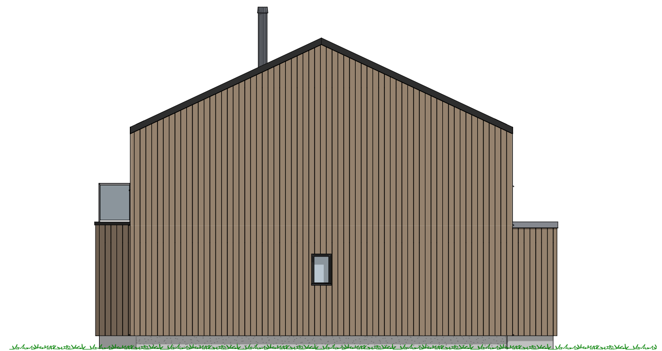
1:100 Fasade Vest
