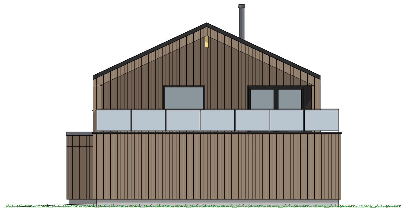
1:100 Fasade Øst
