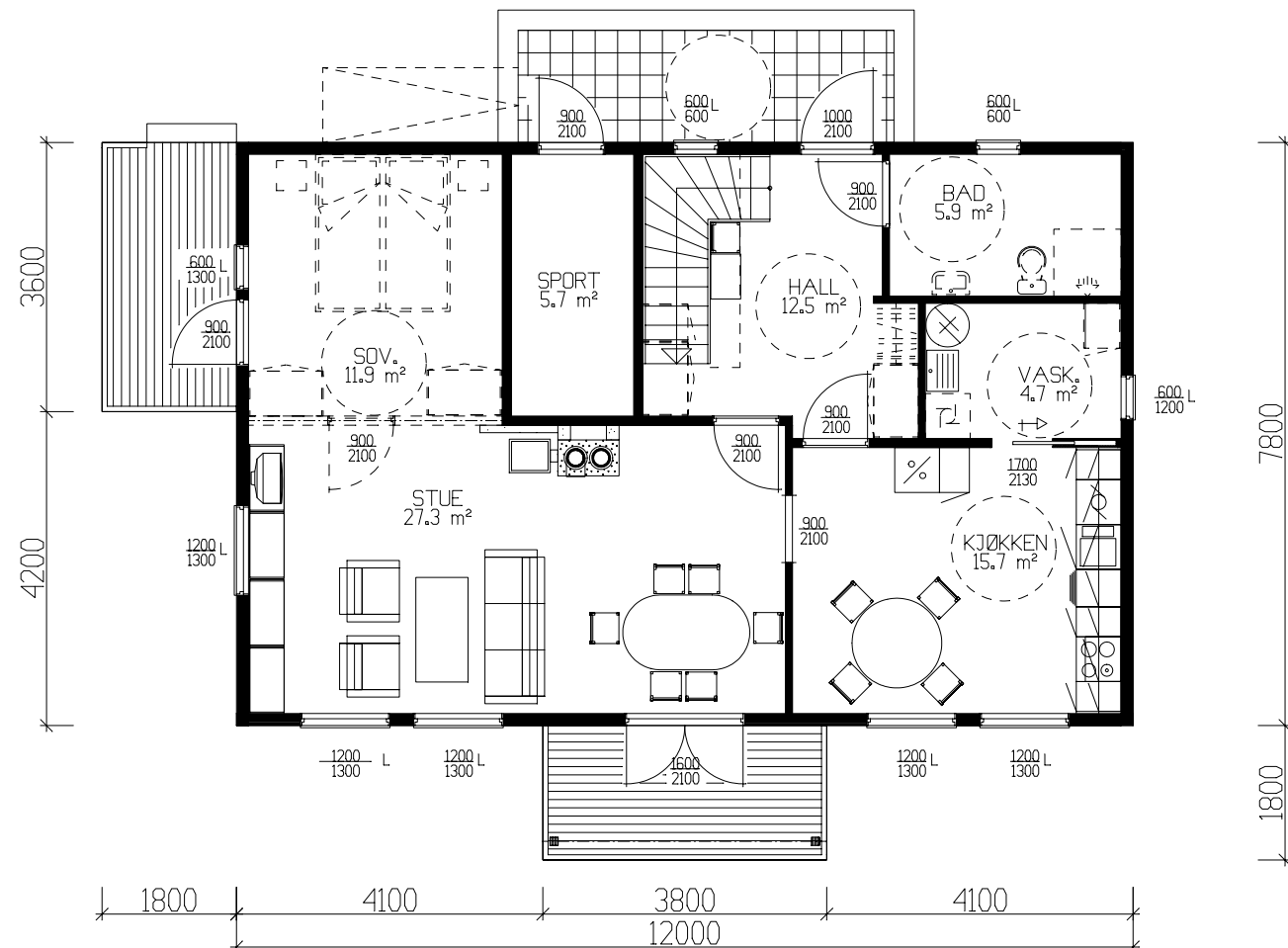
HOVEDPLAN 81.6m² BRA-K + SPORT 5.7m² BRA
