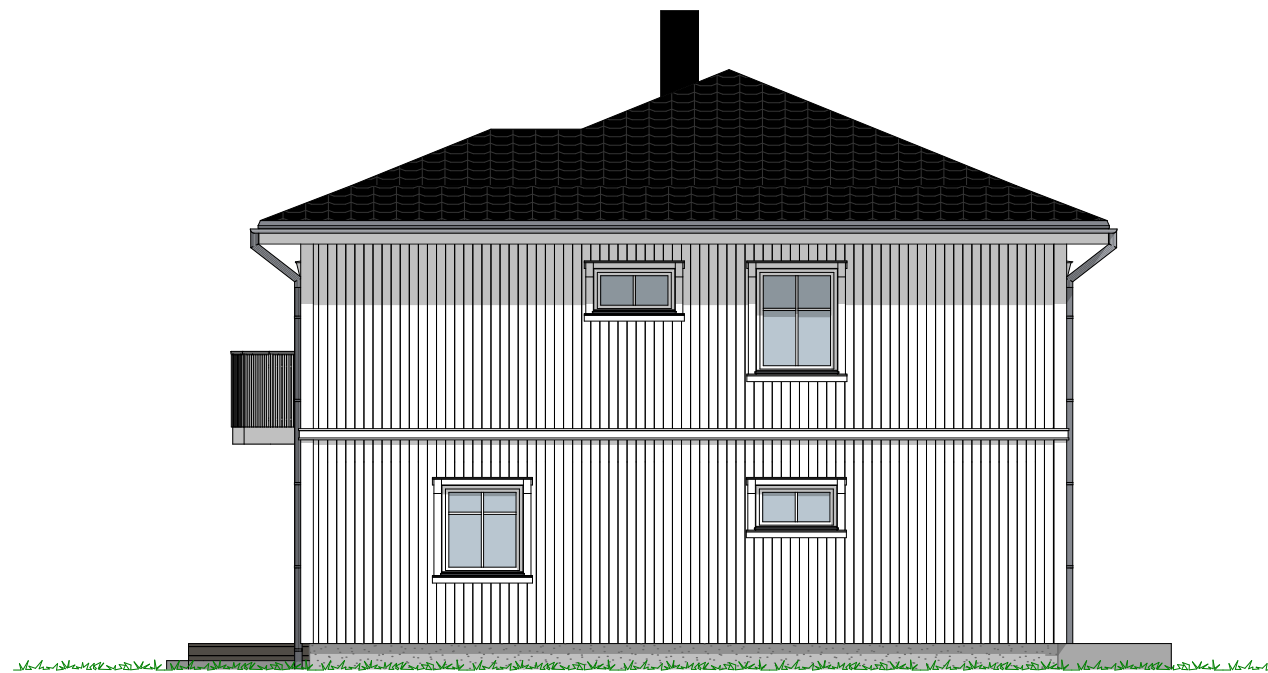
1:100 Fasade Øst
