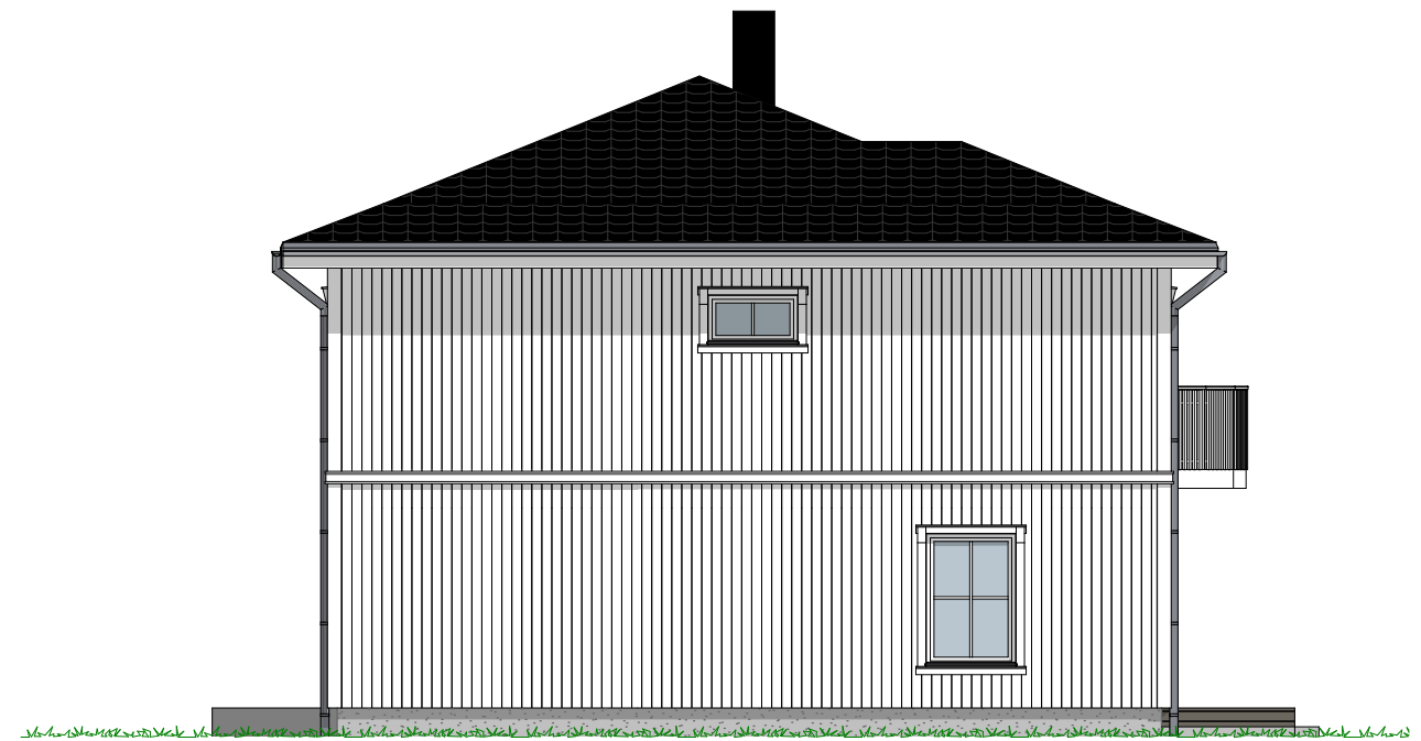
1:100 Fasade Vest
