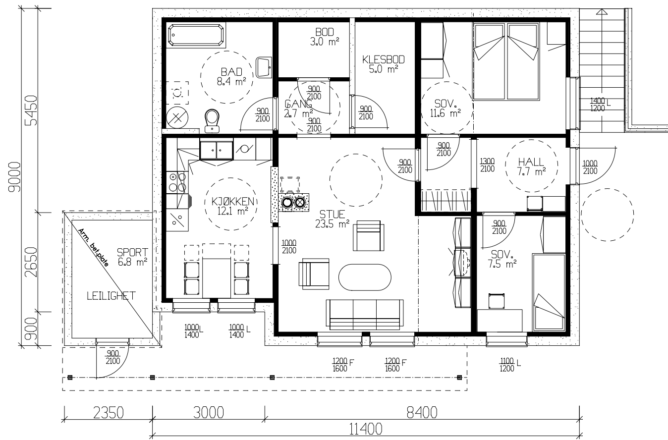
LEILIGHET 85.7m² BRA-K+UTEBOD 6.8m² BRA.
