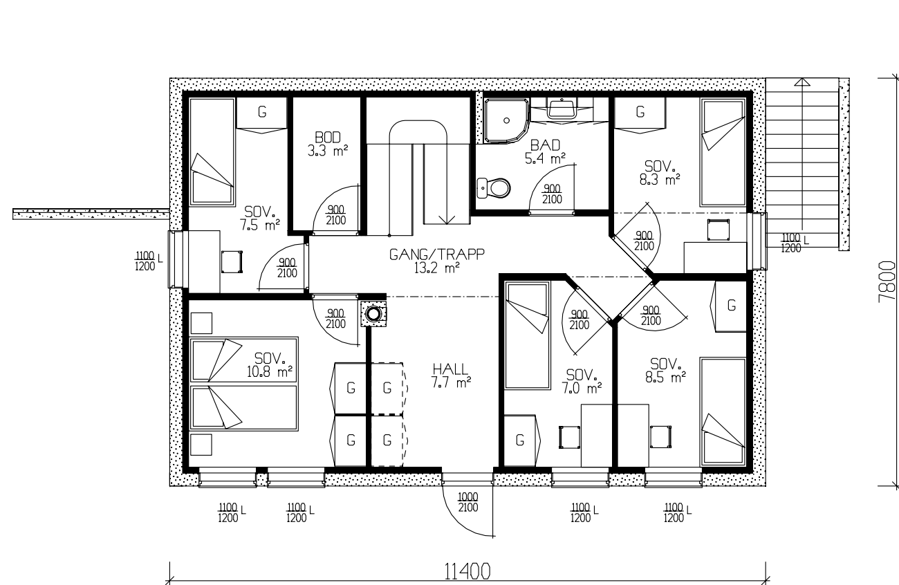
UNDERETASJE 75.6m² BRA.
