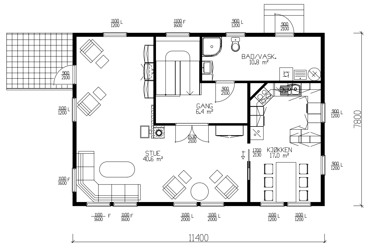
HOVEDPLAN 82.9m² BRA.
