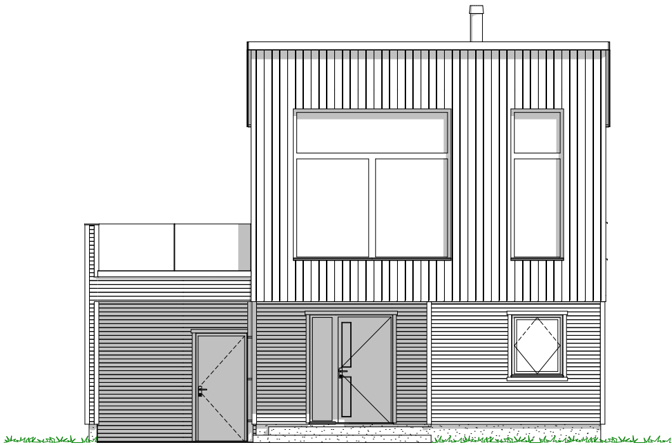
1:100 Fasade Sør Øst
