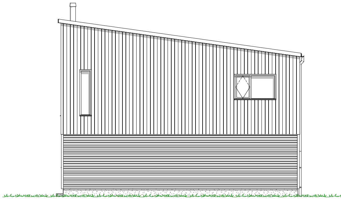
1:100 Fasade Nord Øst
