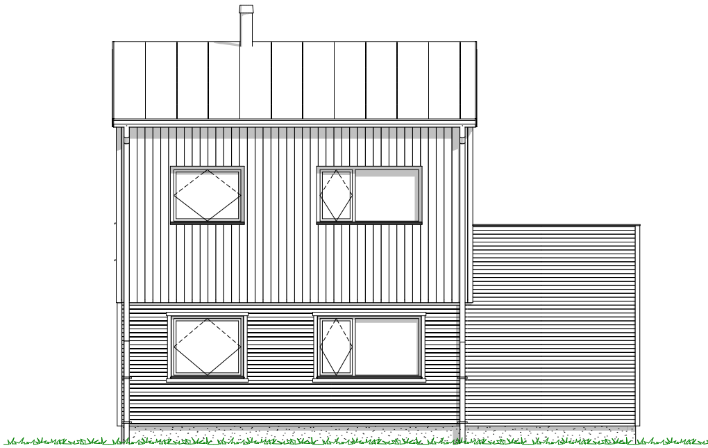
1:100 Fasade Nord Vest
