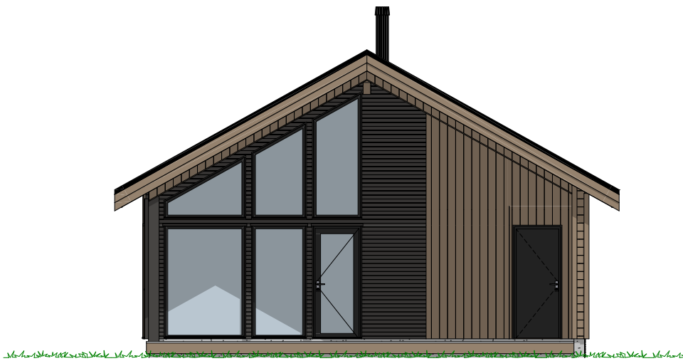
1:100 Fasade Vest
