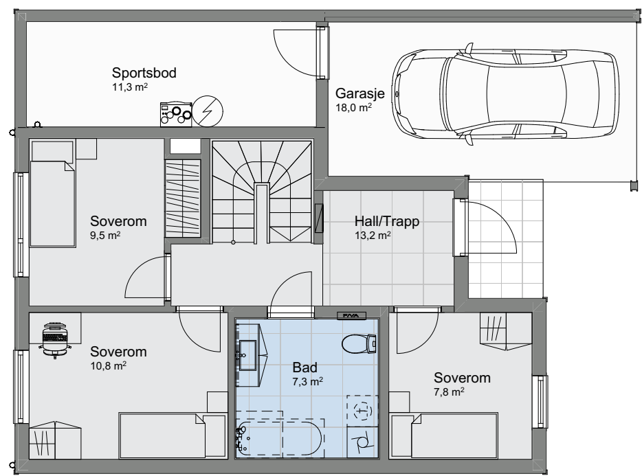
1:100 H. etasje
