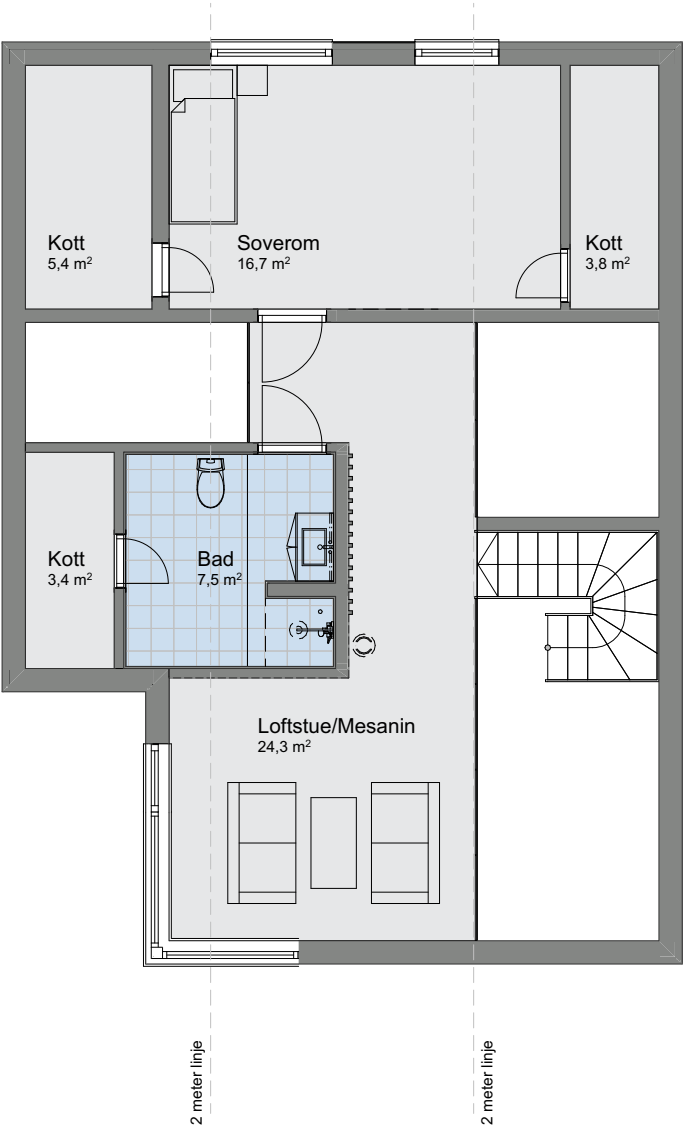
1:100 2. etasje
