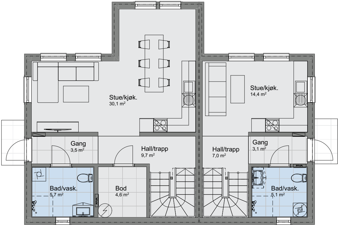
1:100 H. etasje
