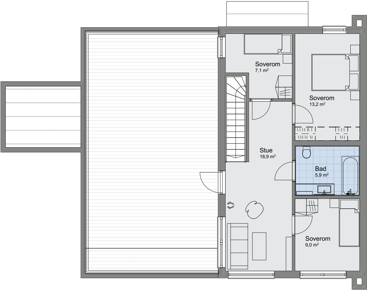
1:100 2. etasje
