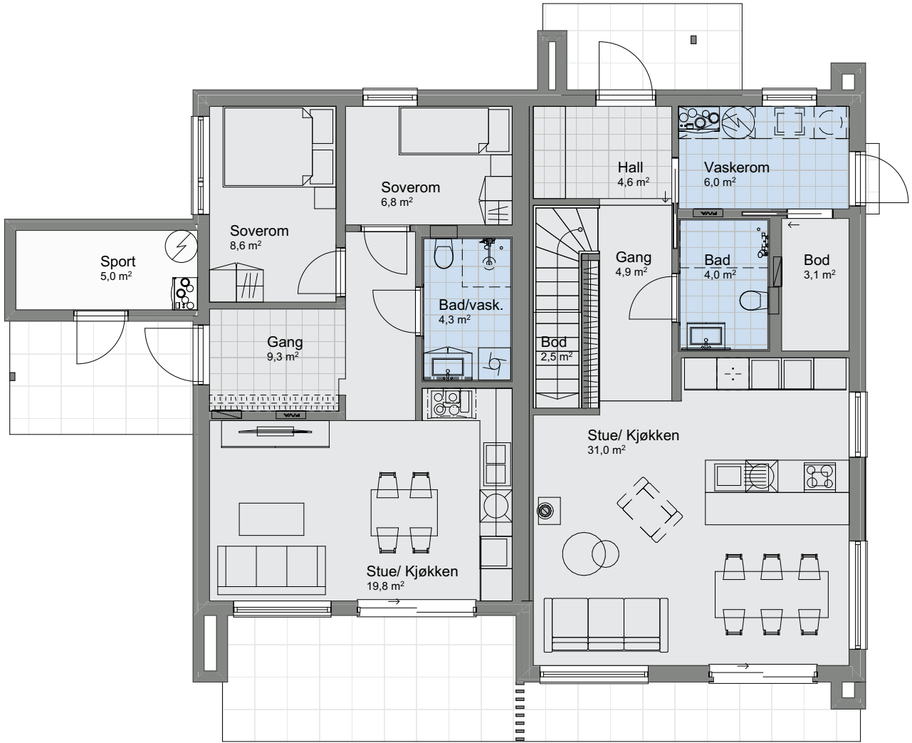
1:100 H. etasje
