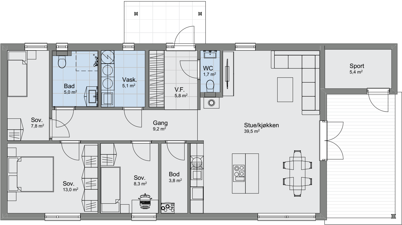
1:100 H. etasje
