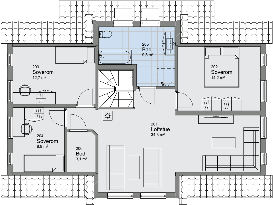
1:100 2. etasje
