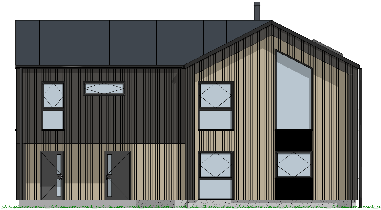
1:100 Fasade Vest
