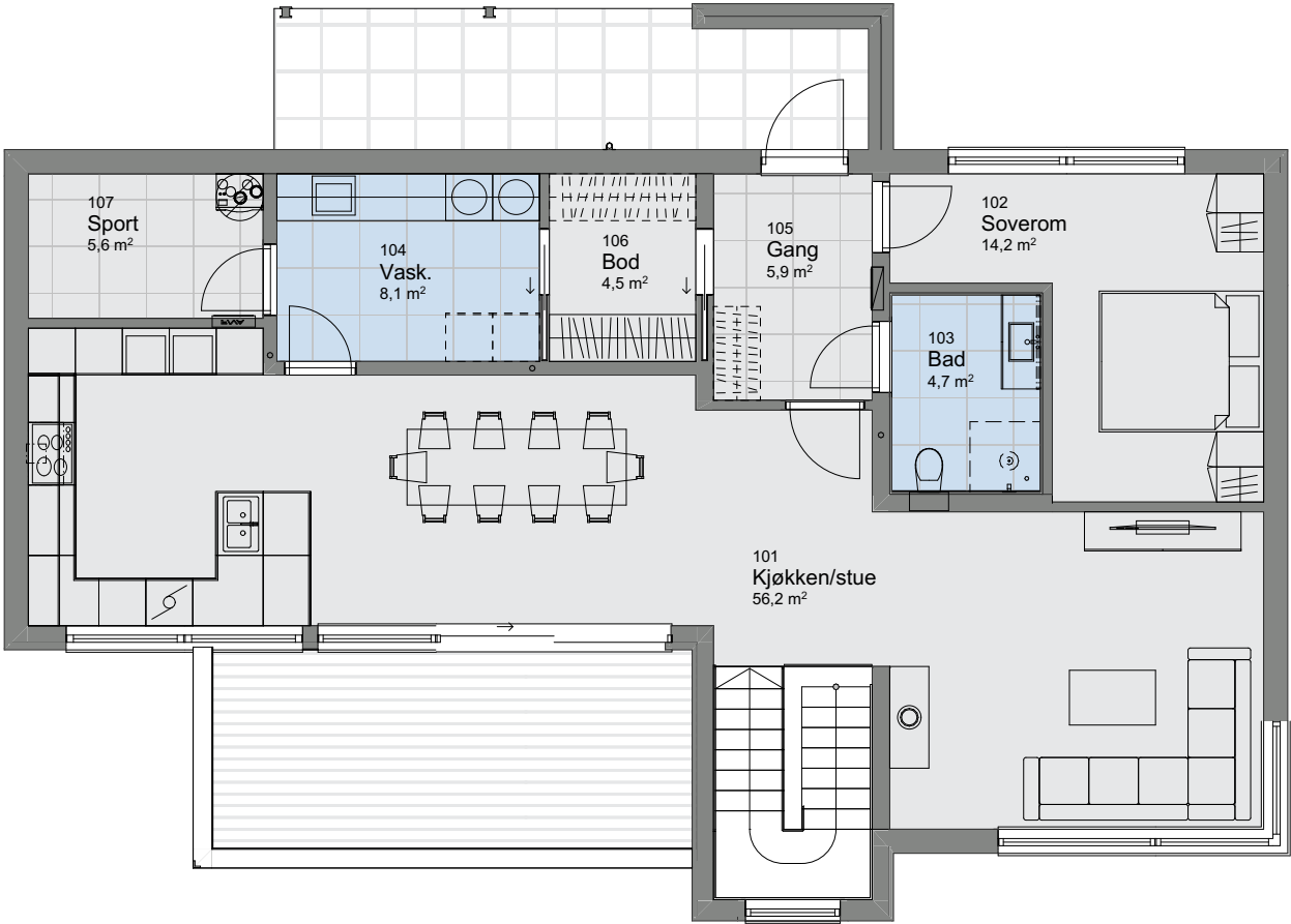
1:100 H. etasje
