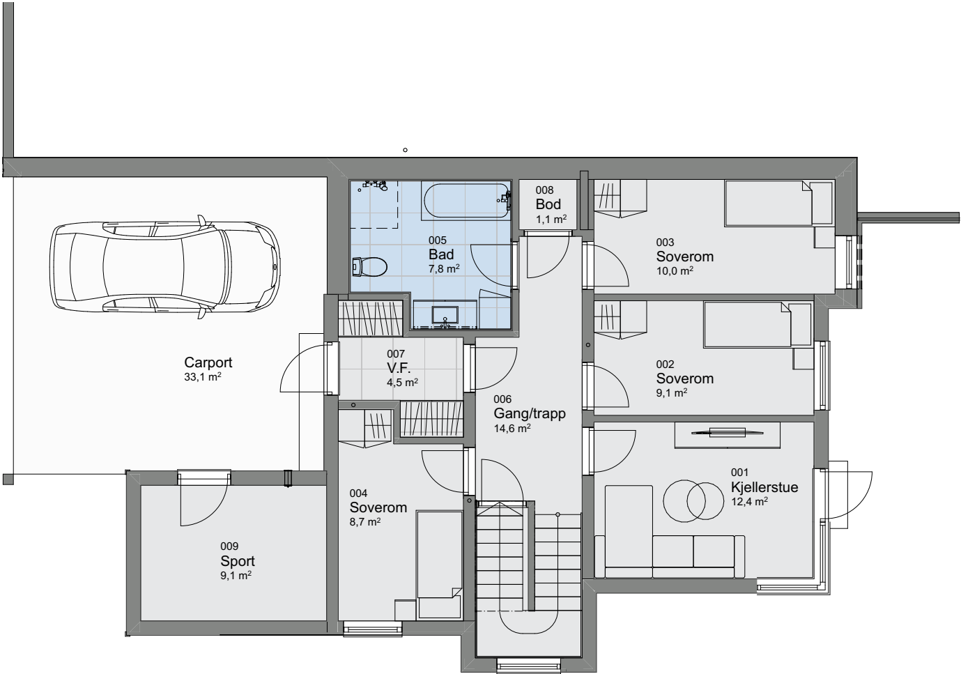
1:100 U. etasje
