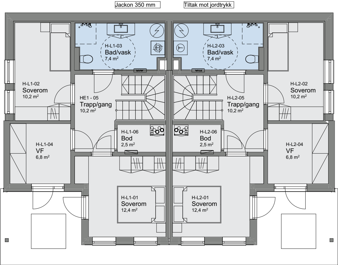
1:100 U. etasje
