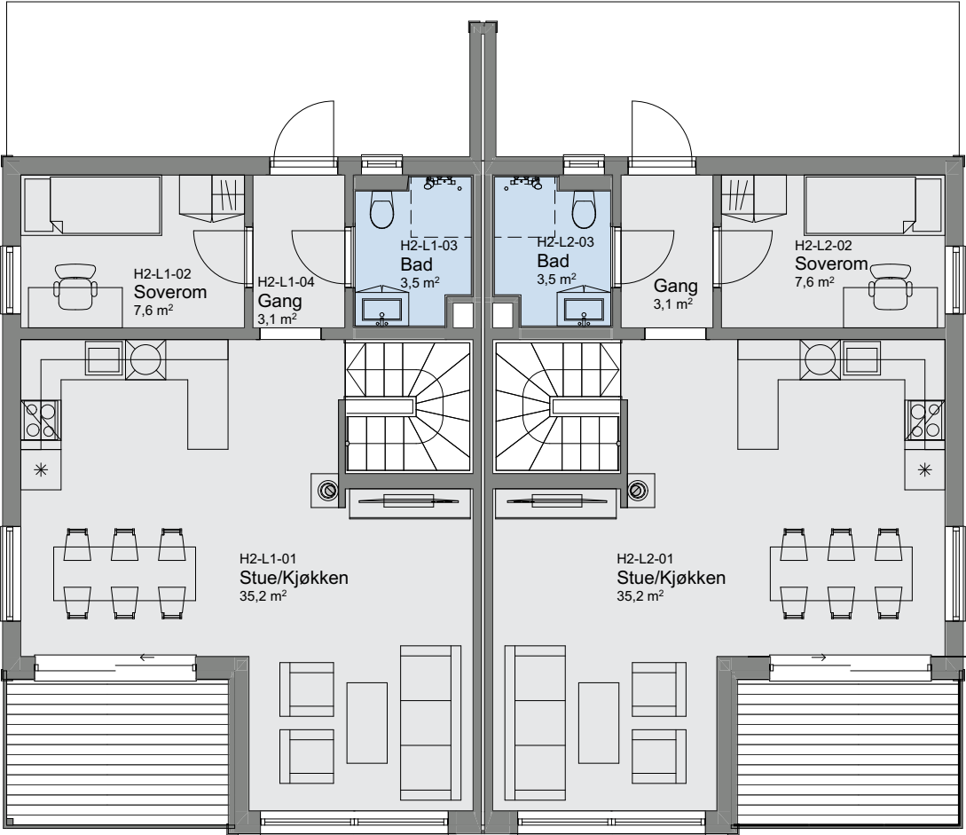
1:100 H. etasje
