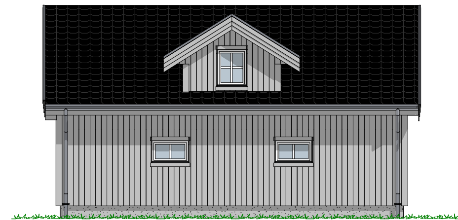
1:100 Fasade Nord Øst
