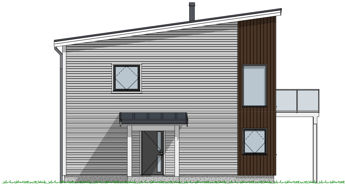
1:100 Fasade VSV
