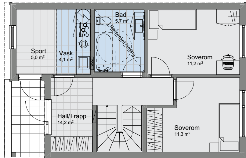
1:100 H. etasje
