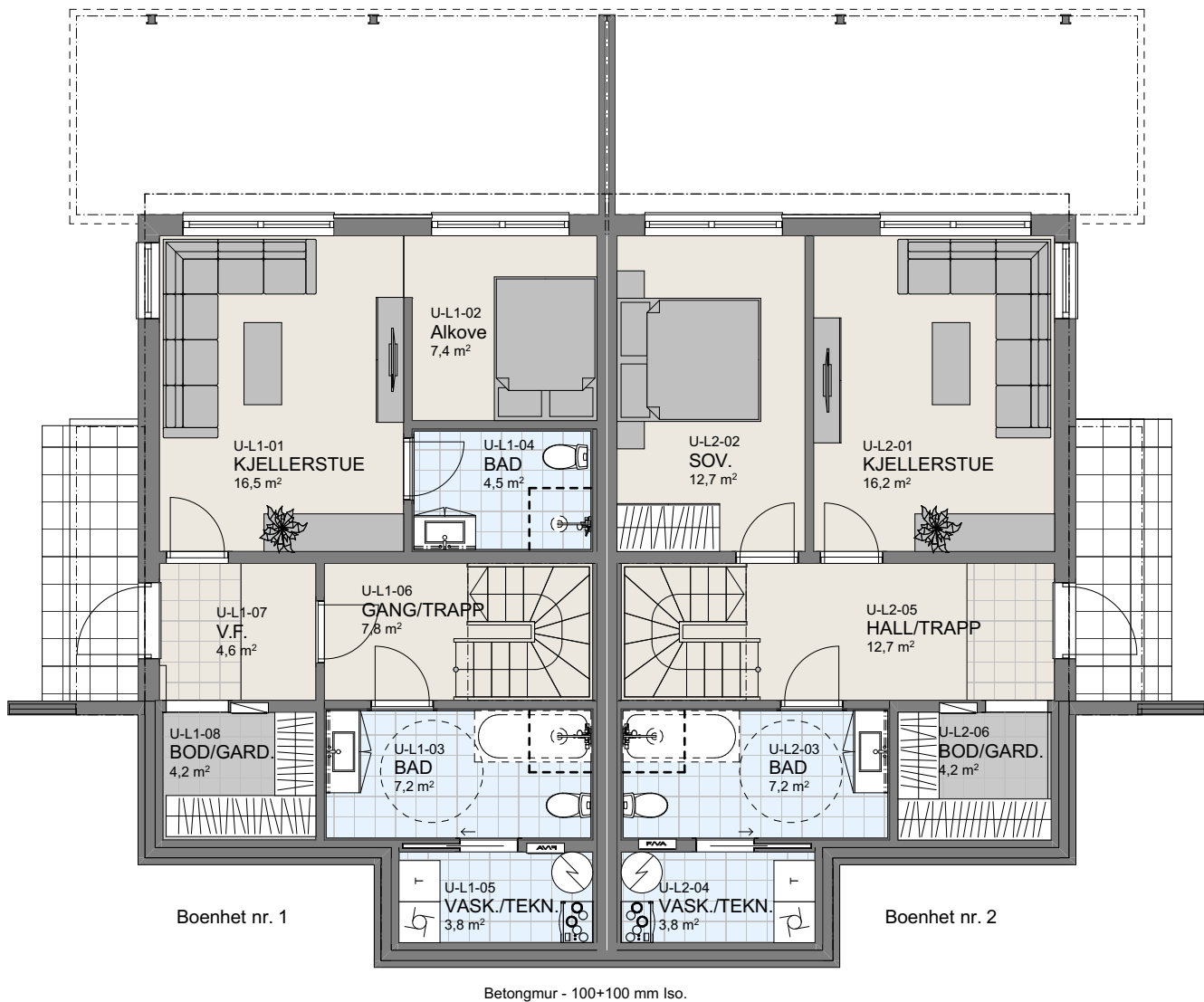
1:100 U. Etasje
