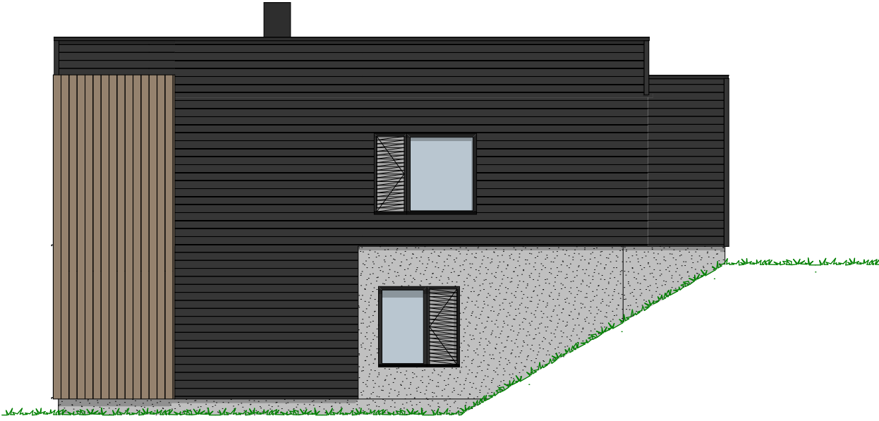
1:100 Fasade Øst
