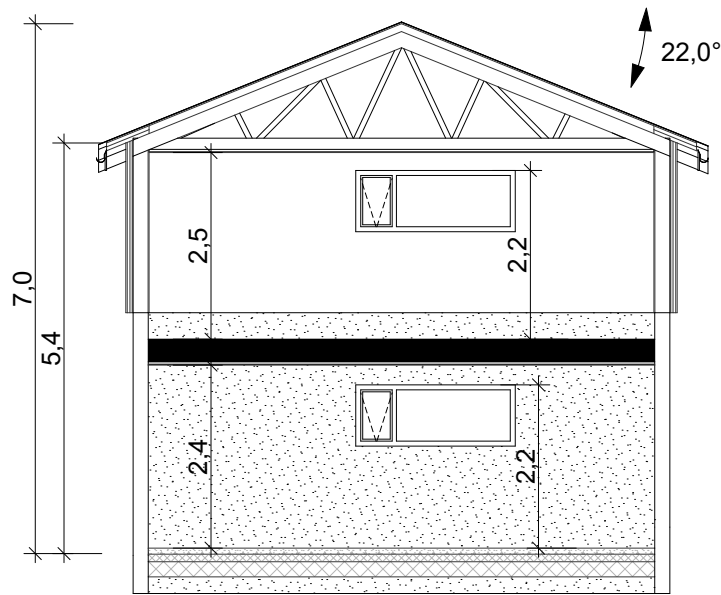
1:100 Snitt B
