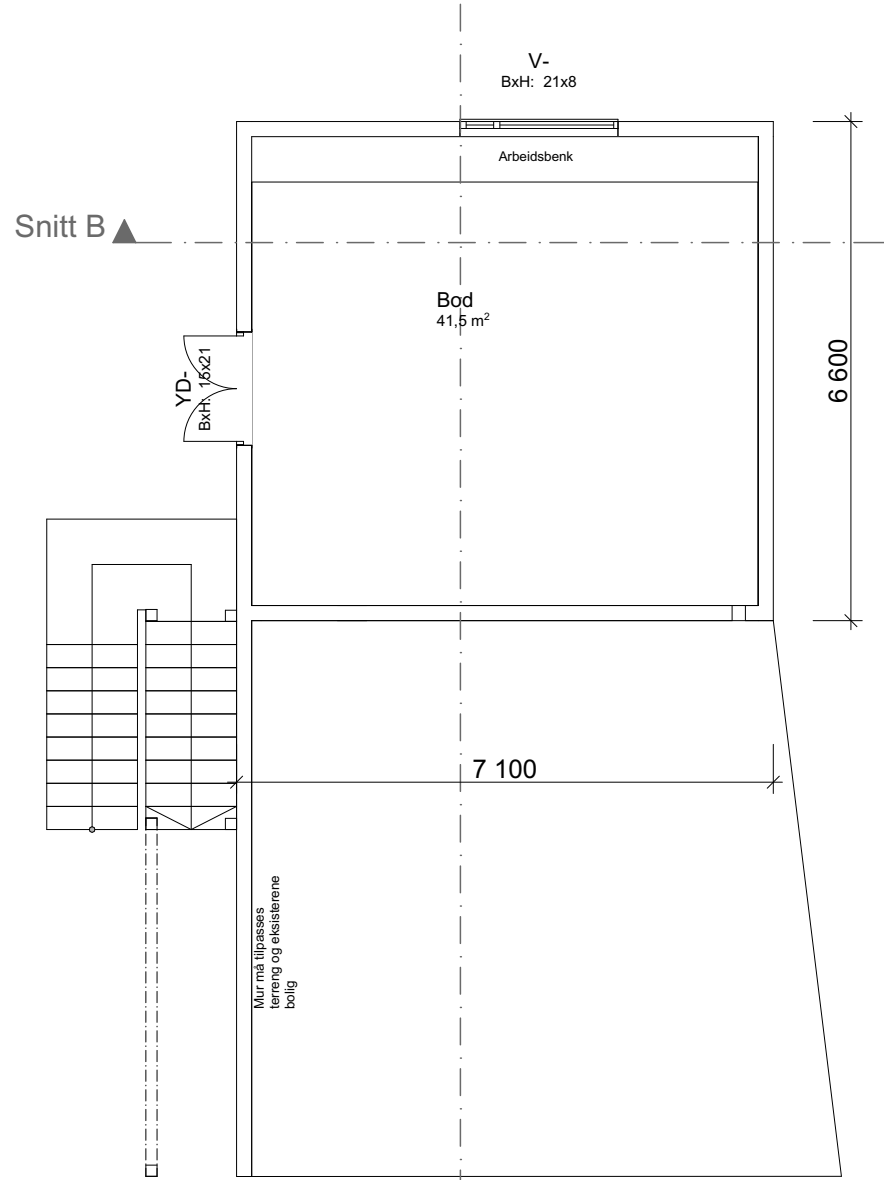
1:100 U. etasje
