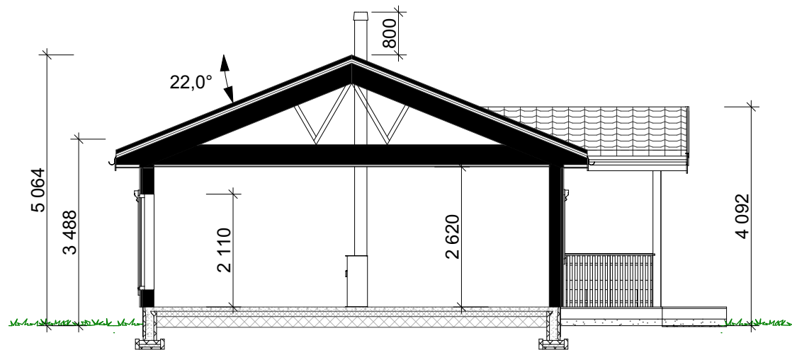
1:100 Snitt A
