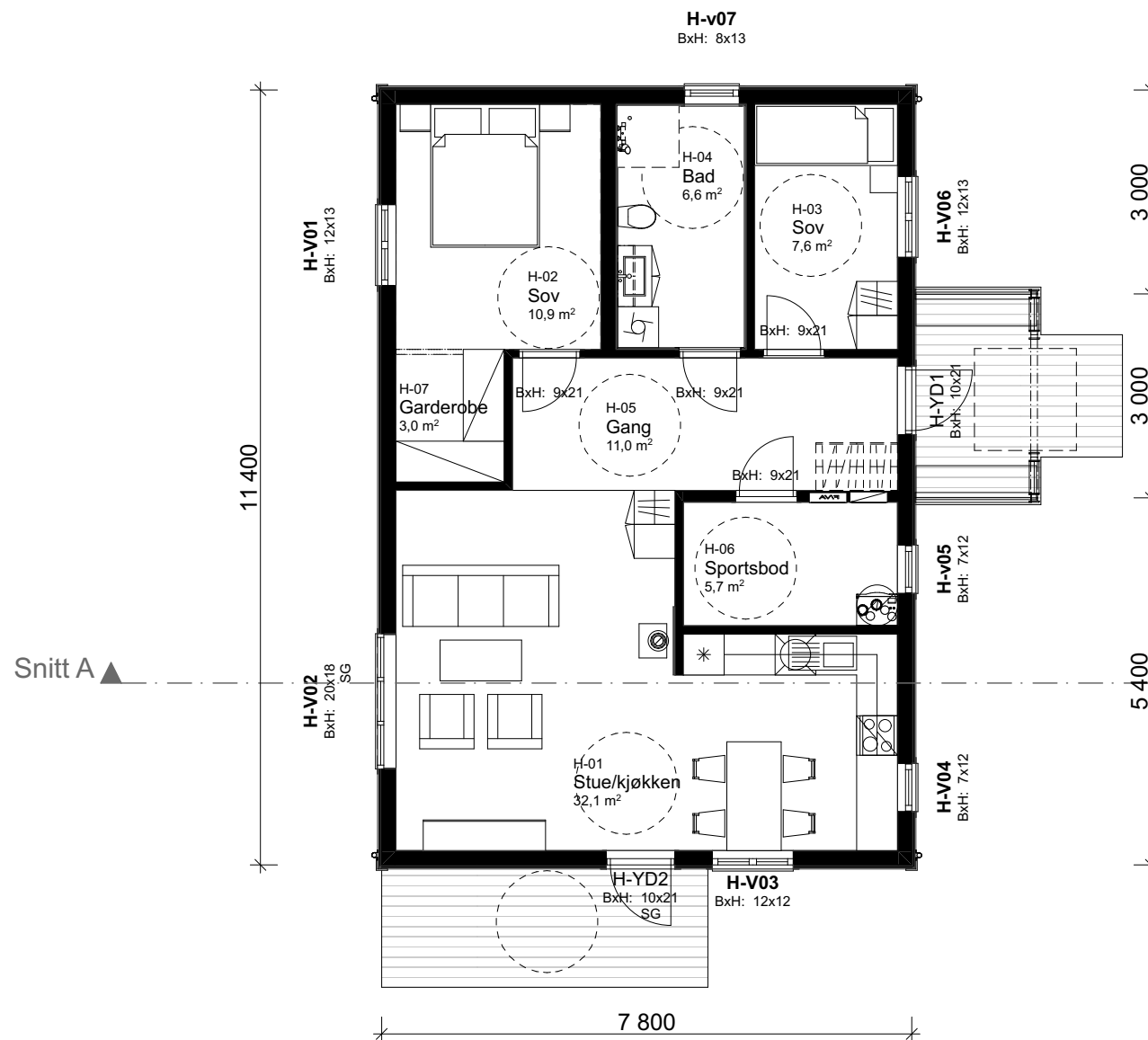
1:100 H. etasje
