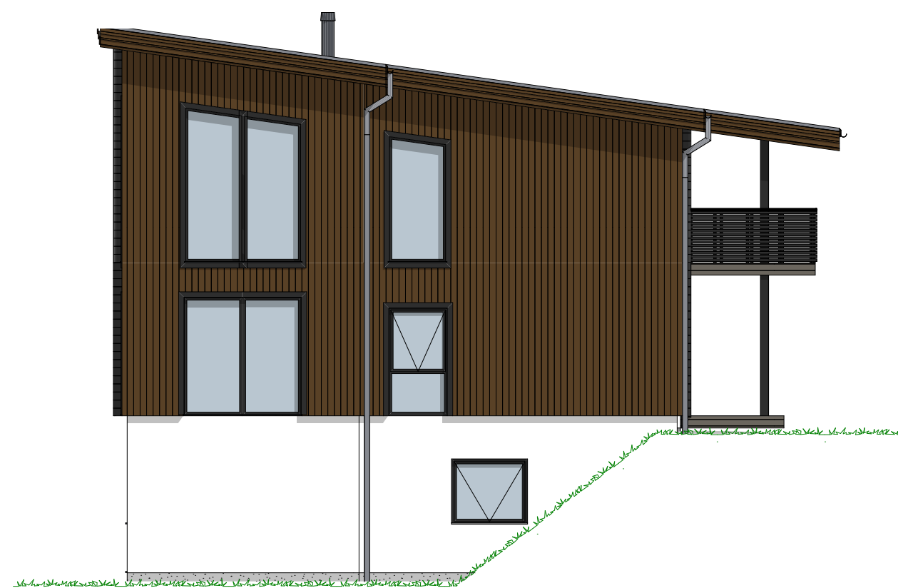
1:100 Fasade Øst
