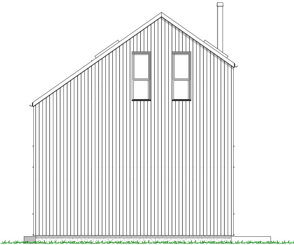
1:100 Fasade Nord
