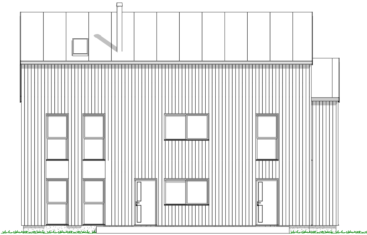
1:100 Fasade Vest
