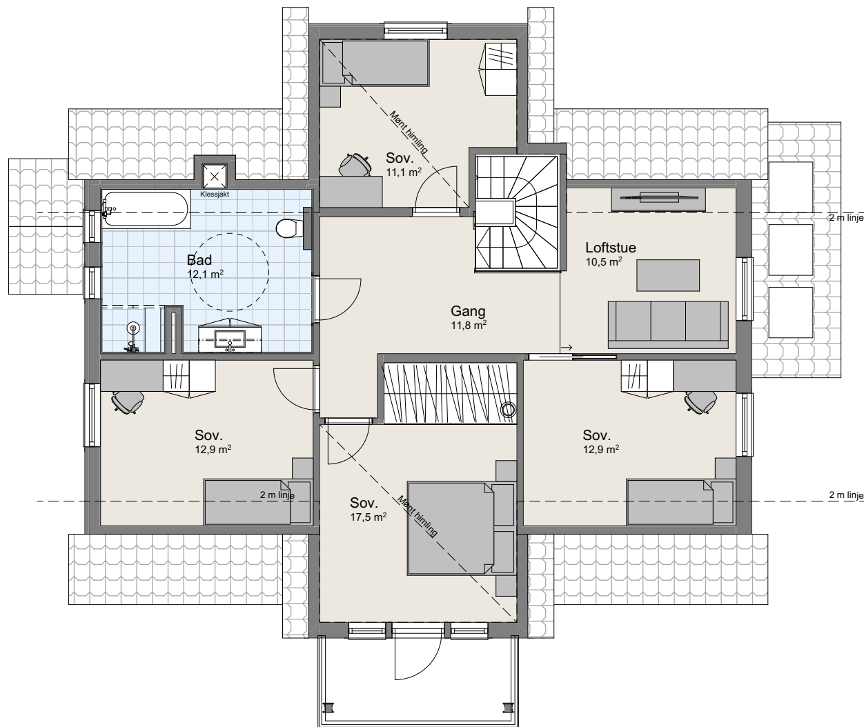
1:100 2.Etasje
