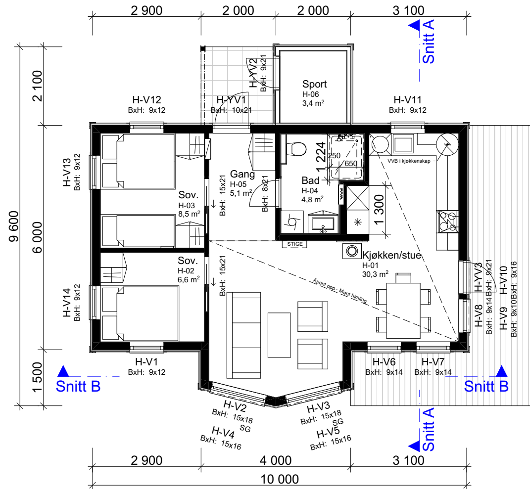
1:100 H. Etasje
