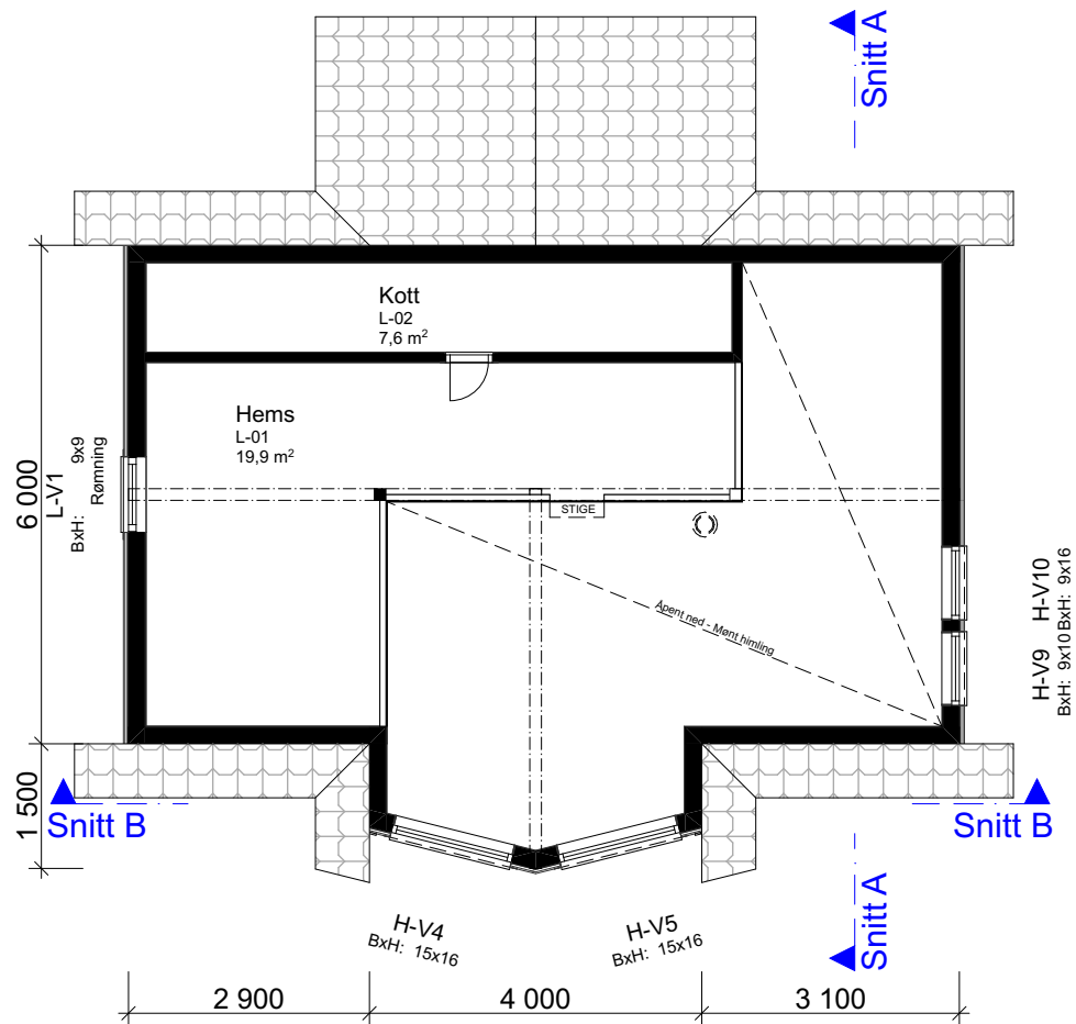
1:100 2.Etasje
