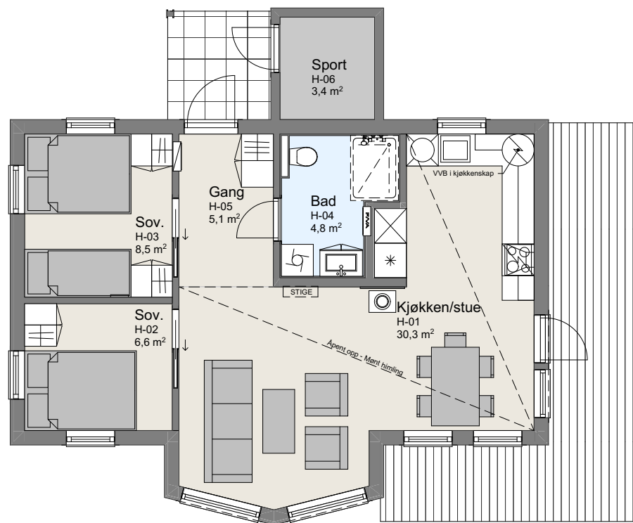
1:100 H. Etasje
